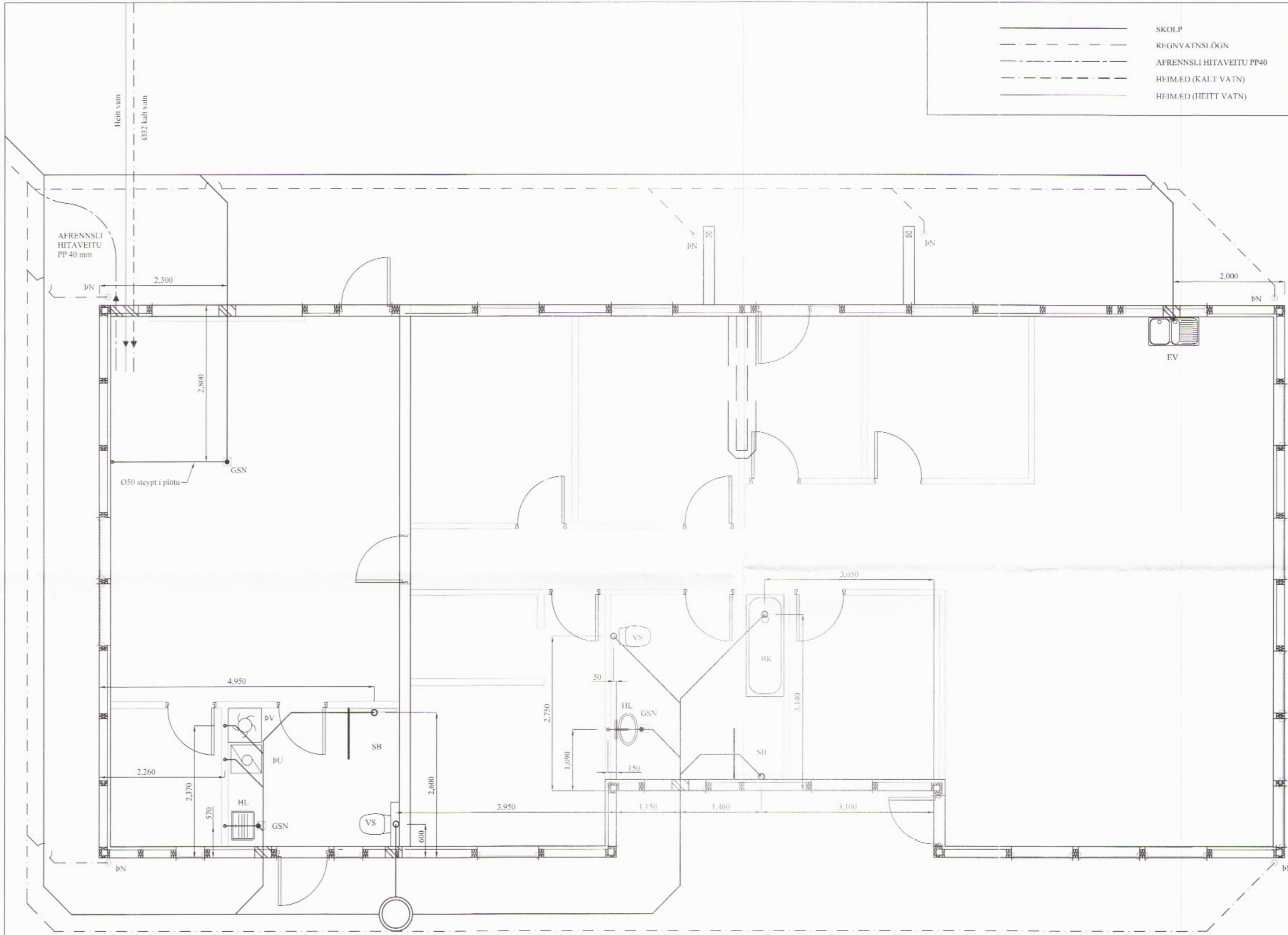
Grunnmynd fráveituagna MKV: 1:50
