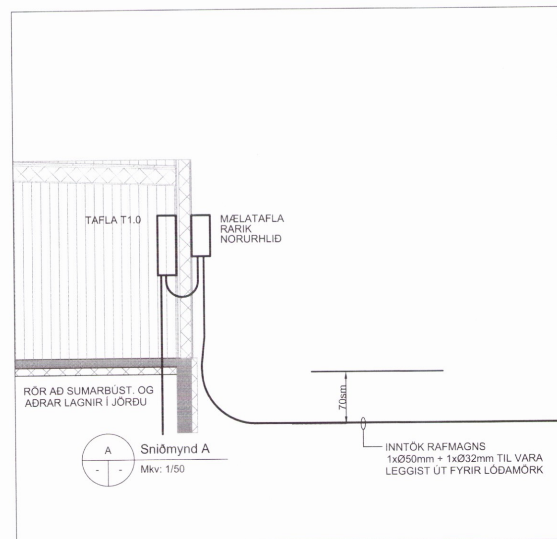
SNÍÐMYND 1:50
