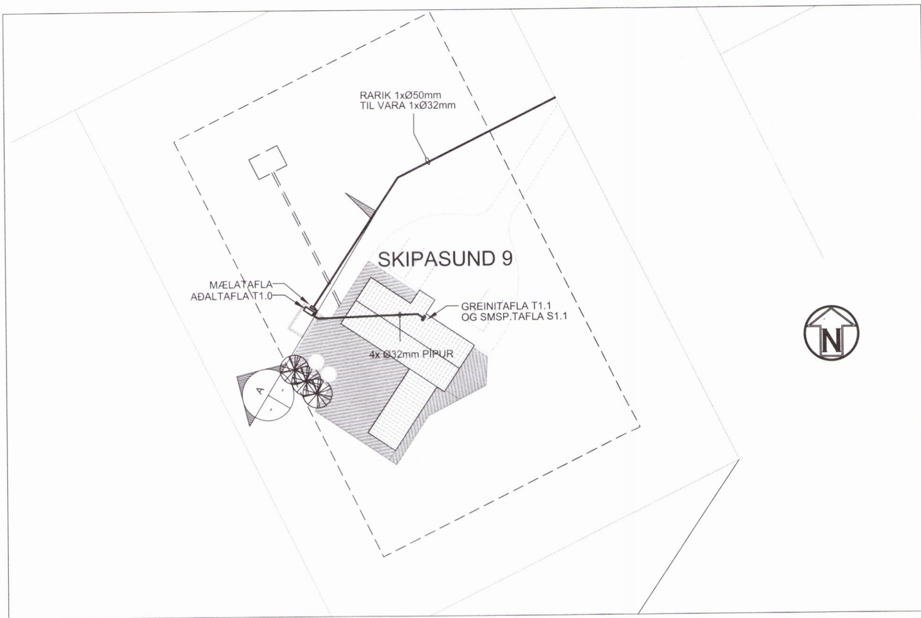
AFSTÖÐUMYND 1:500
