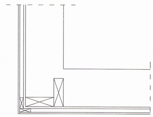
FRÁGANGUR HORNS MKV. 1:20
