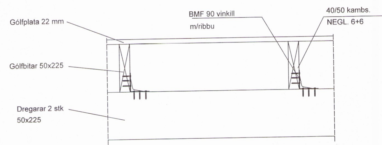
Festing dregarar/gólfbitar 1:10
