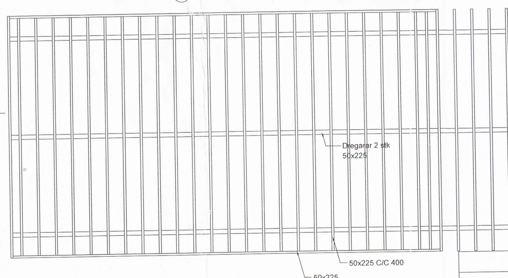
Gólf 1:50
