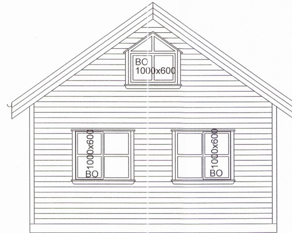
Hlið 2 (Norður) 1:50
