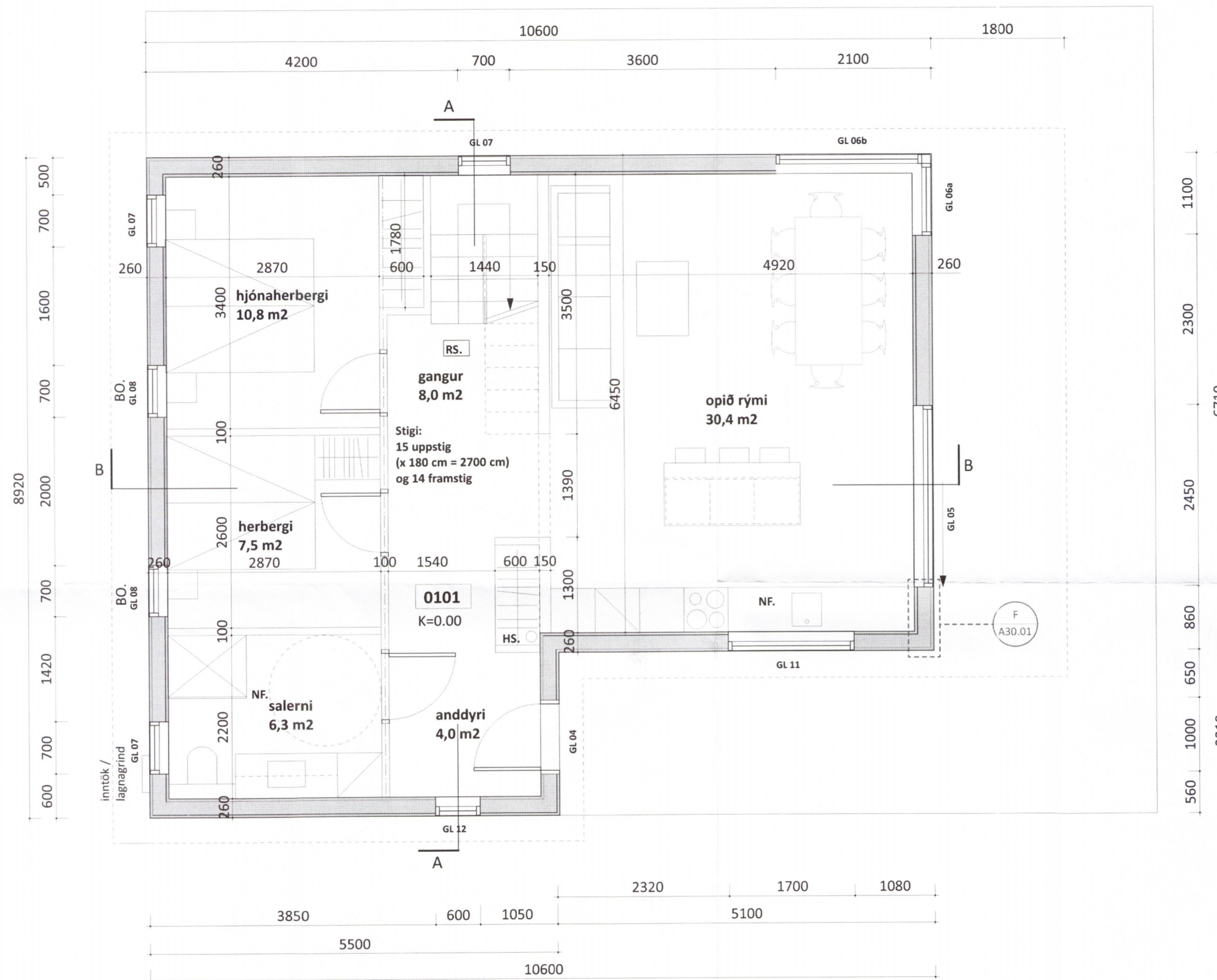
GRUNNMYND 1. HÆÐ, M.KV. 1:50
