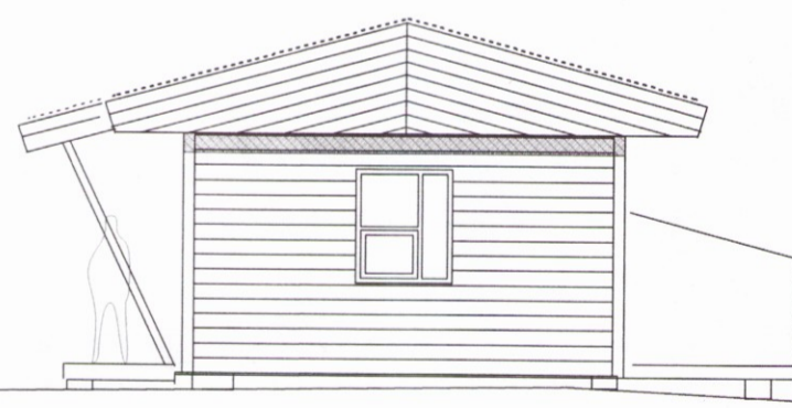
NORDLÆGUR GAFL
