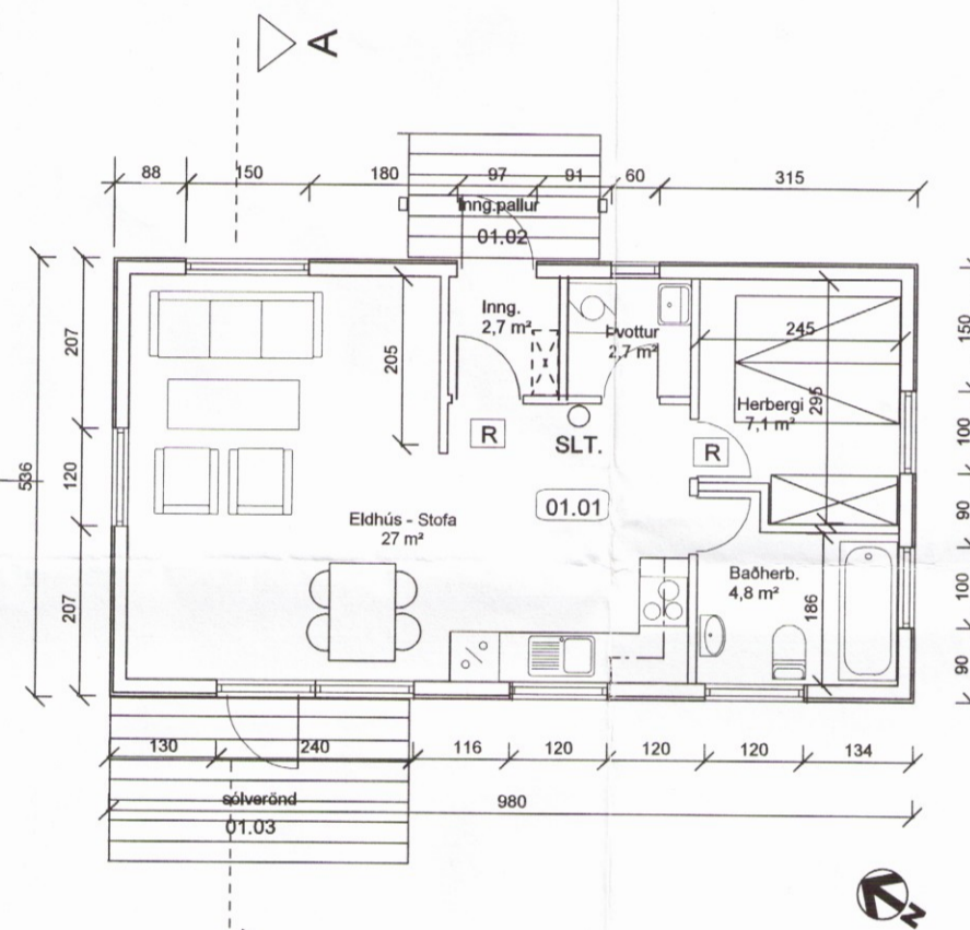
GRUNNMYND mkv. 1: 100
