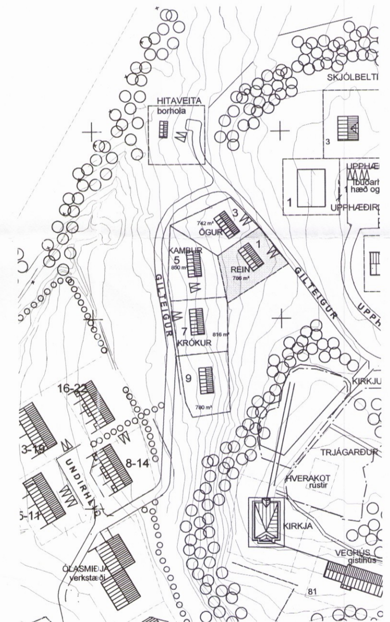
AFSTÖÐUMYNDMYND mkv. 1: 500
