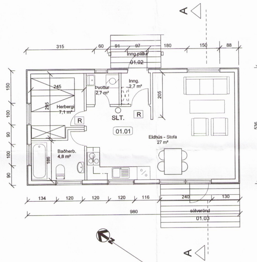
GRUNNMYND mkv. 1: 100
