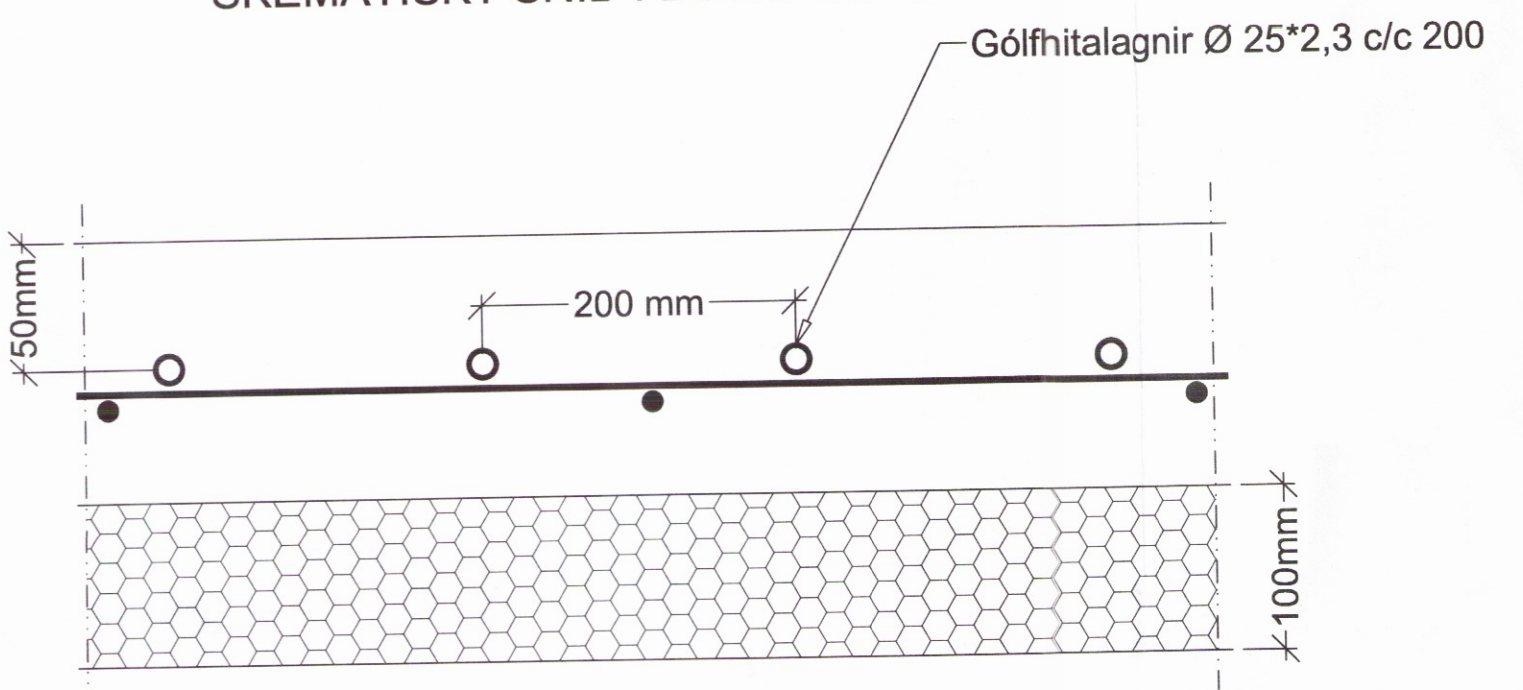
SKEMATISKT SNIÐ Í BOTNPLÖTU
