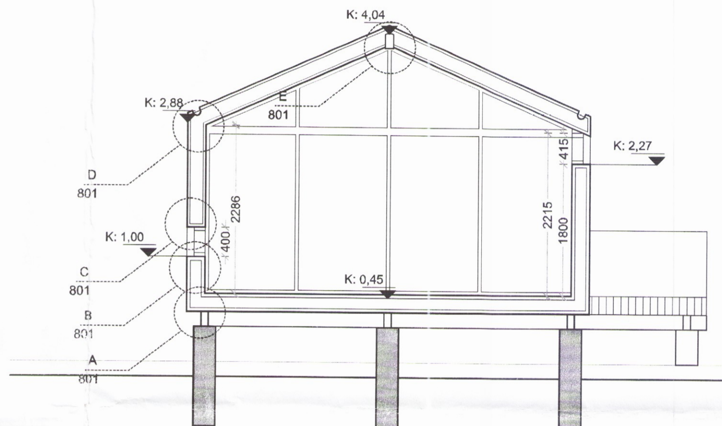
Sneiðing A-A MKV 1:50
