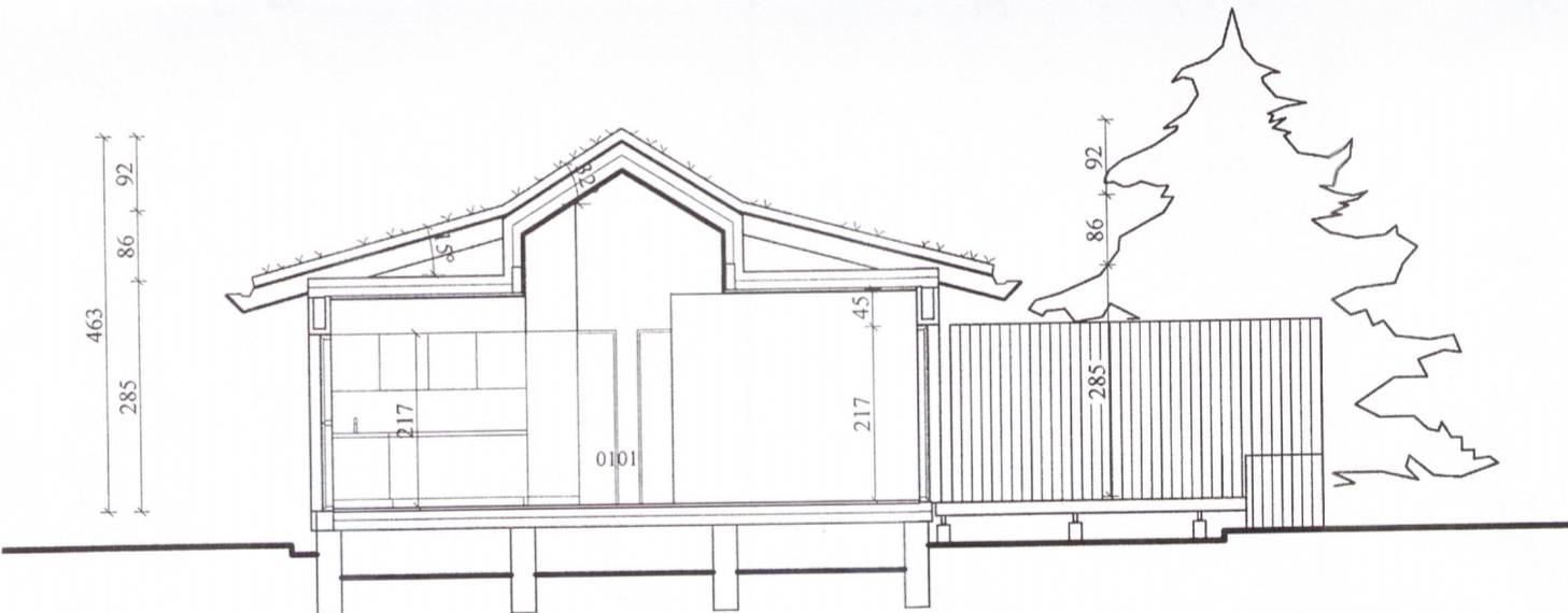
Snið A-A
