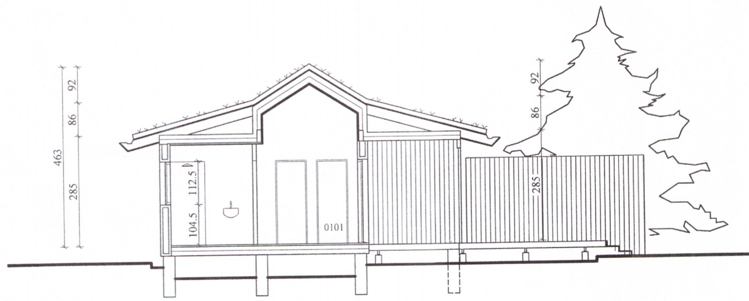
Snið B-B
