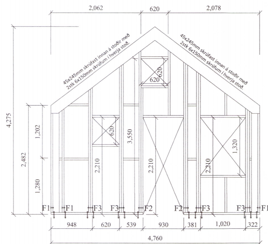
Grind nr. 1 - 45x145mm grindaefni
