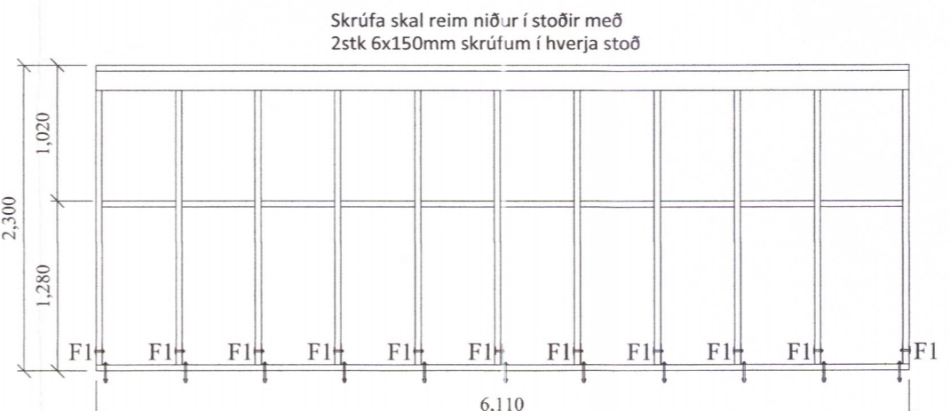
Grind nr. 4 - 45x145mm grindaefni
