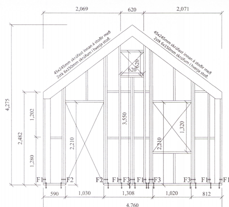
Grind nr. 3 - 45x145mm grindaefni
