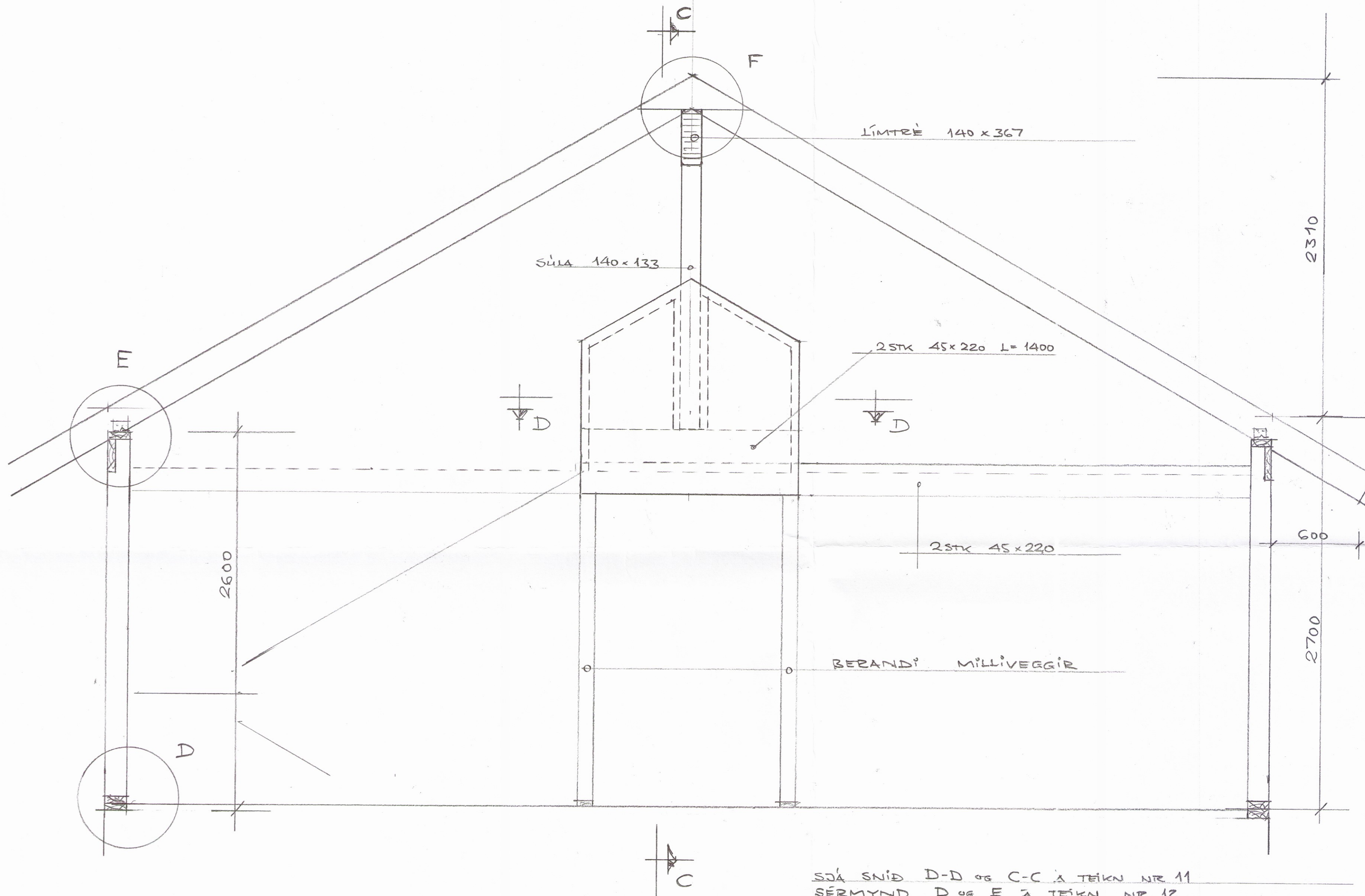
PVERSNID Í MIÐJAN BÚSTAÐ M 1:20
