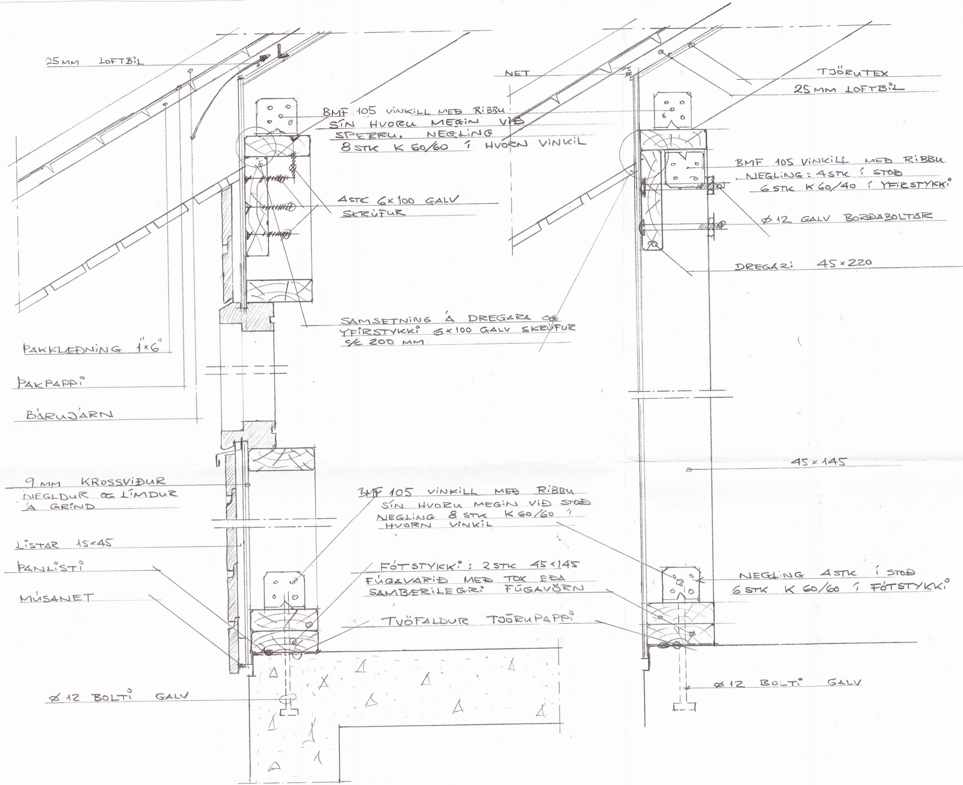
SÉRMYND D 06 E í GLUGGABÍLI M 1:5
