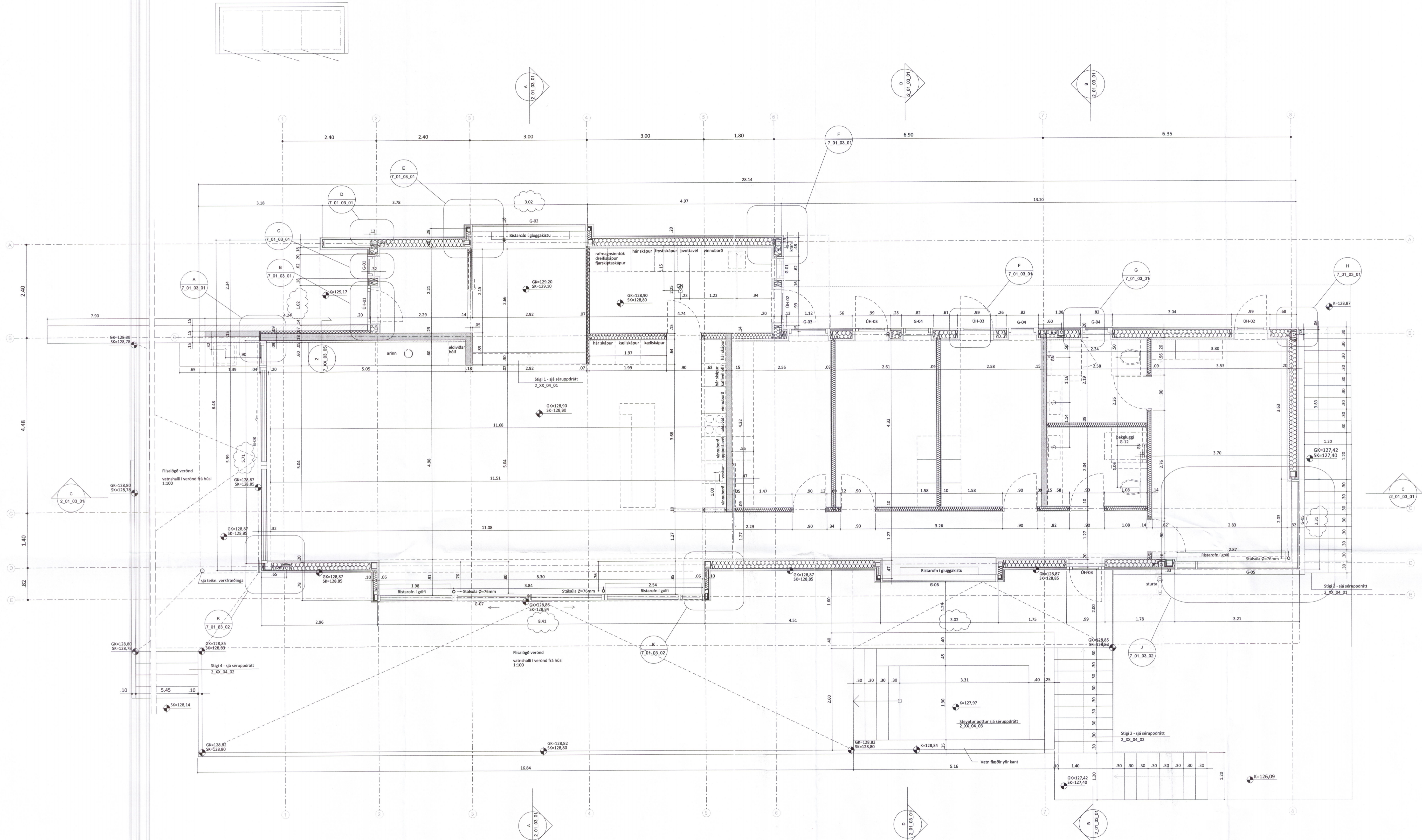
Grunnmynd - 1. hæð
