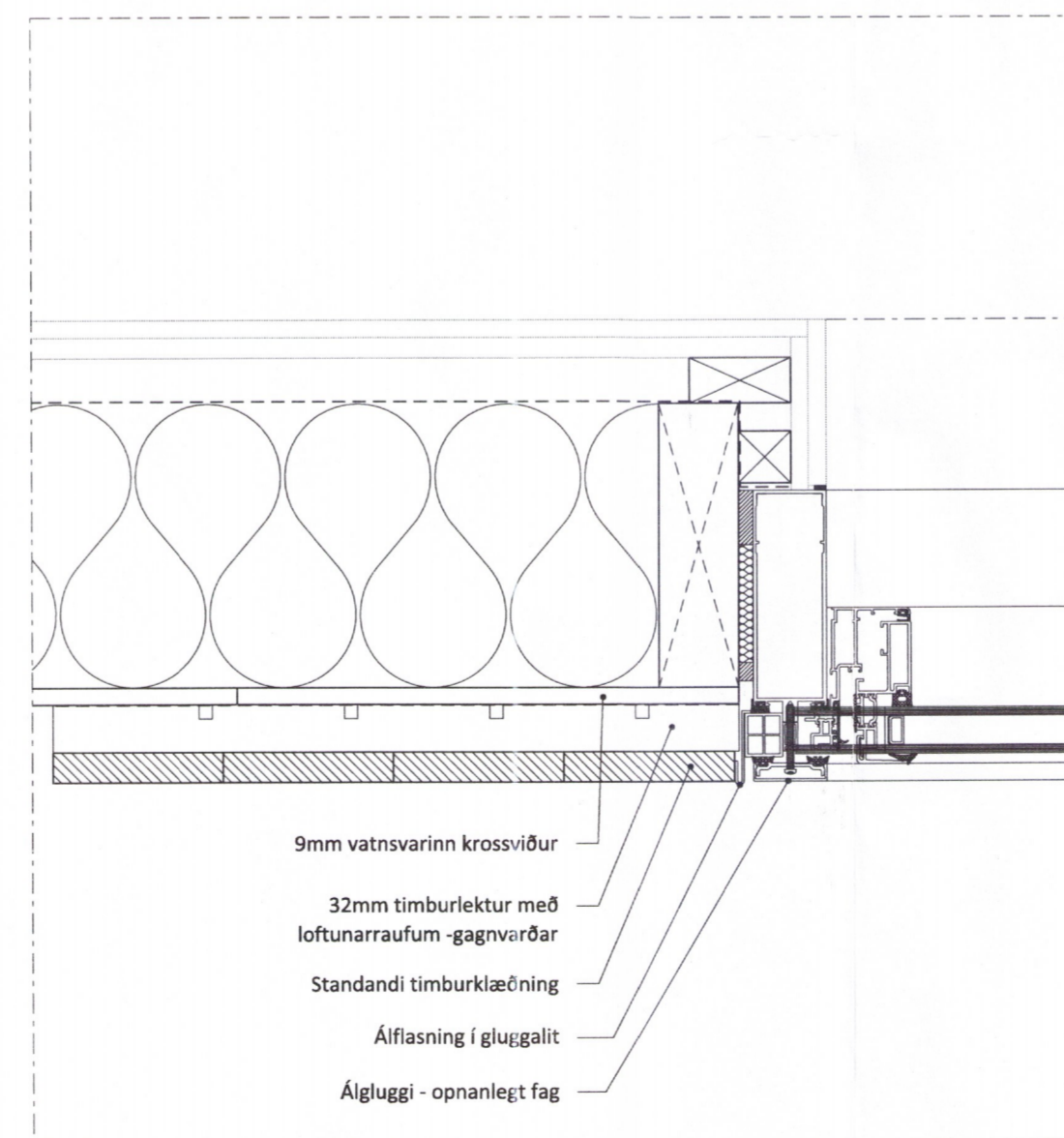
J Hornluggi í hjónaherbergi 2_XX_03_02 Mkv. 1:5
