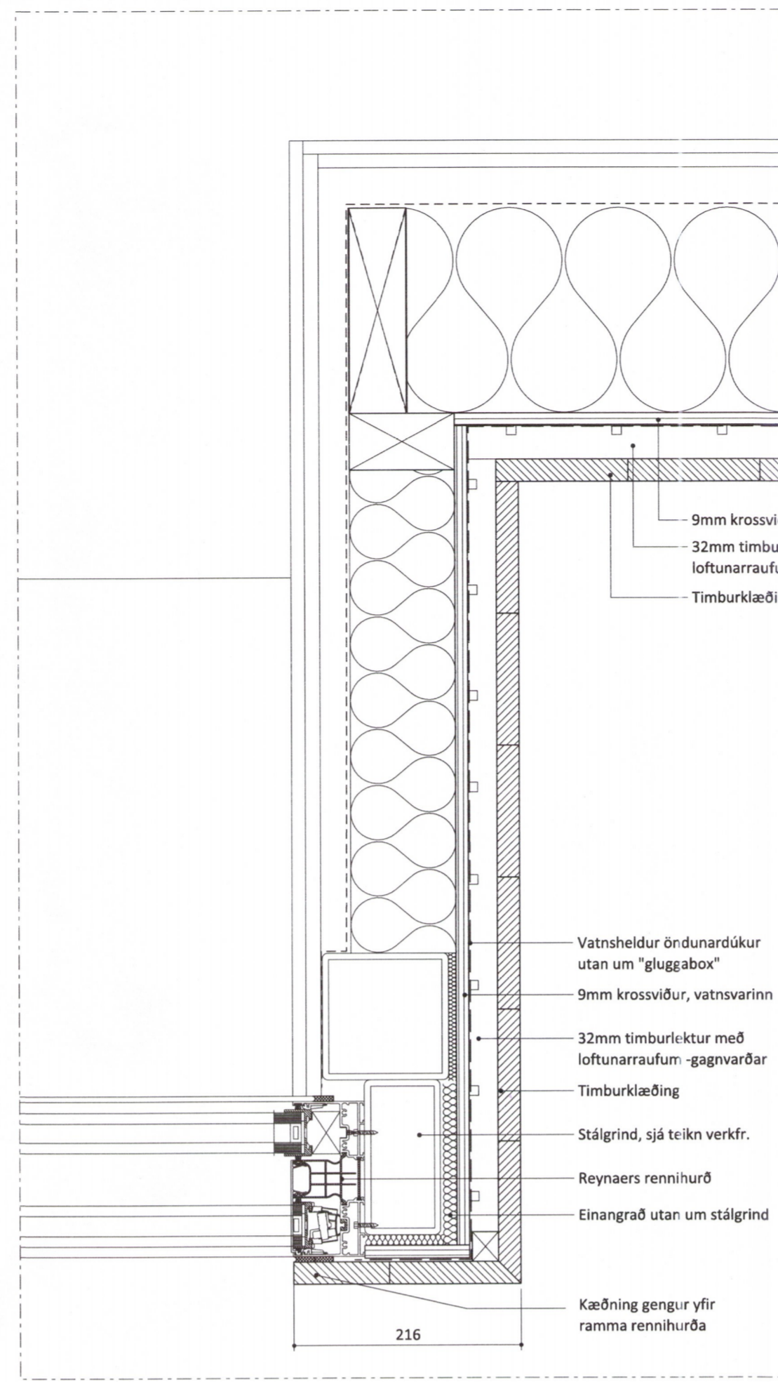
K Gluggabox með rennihurð 2_XX_03_02 Mkv. 1:5
