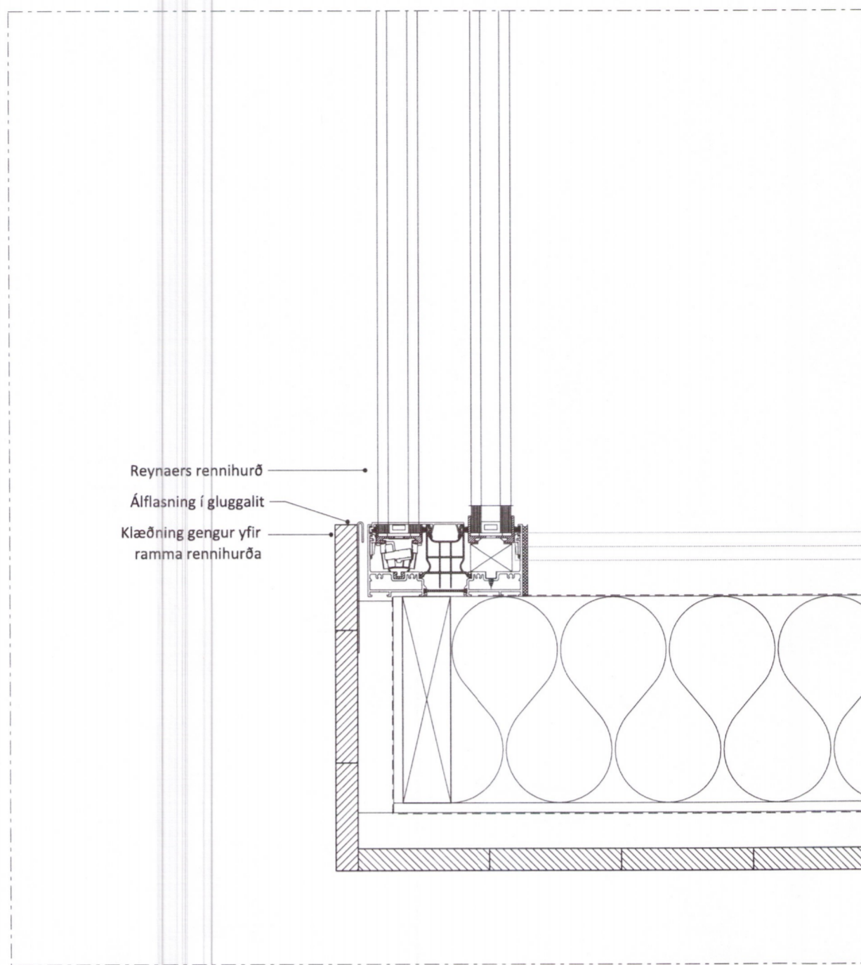
L Rennihurð við úthorn 2_XX_03_02 Mkv. 1:5
