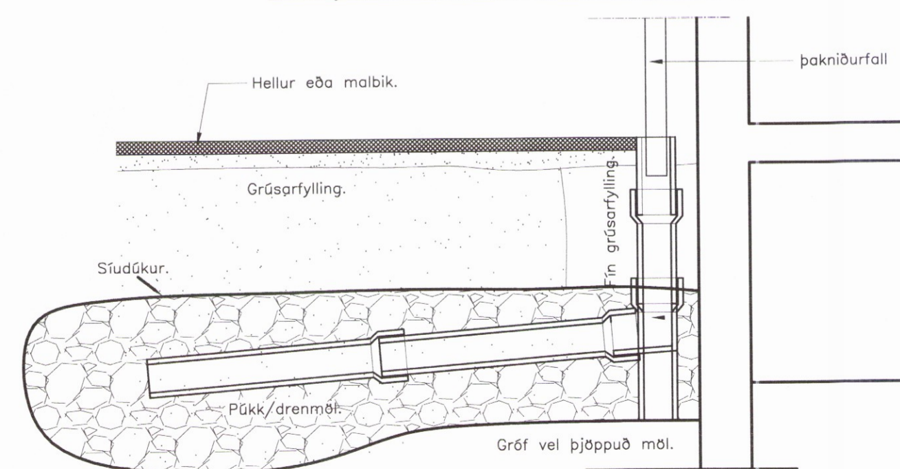
Sérmynd af þakniðurfalli í jörð. 1:20.
