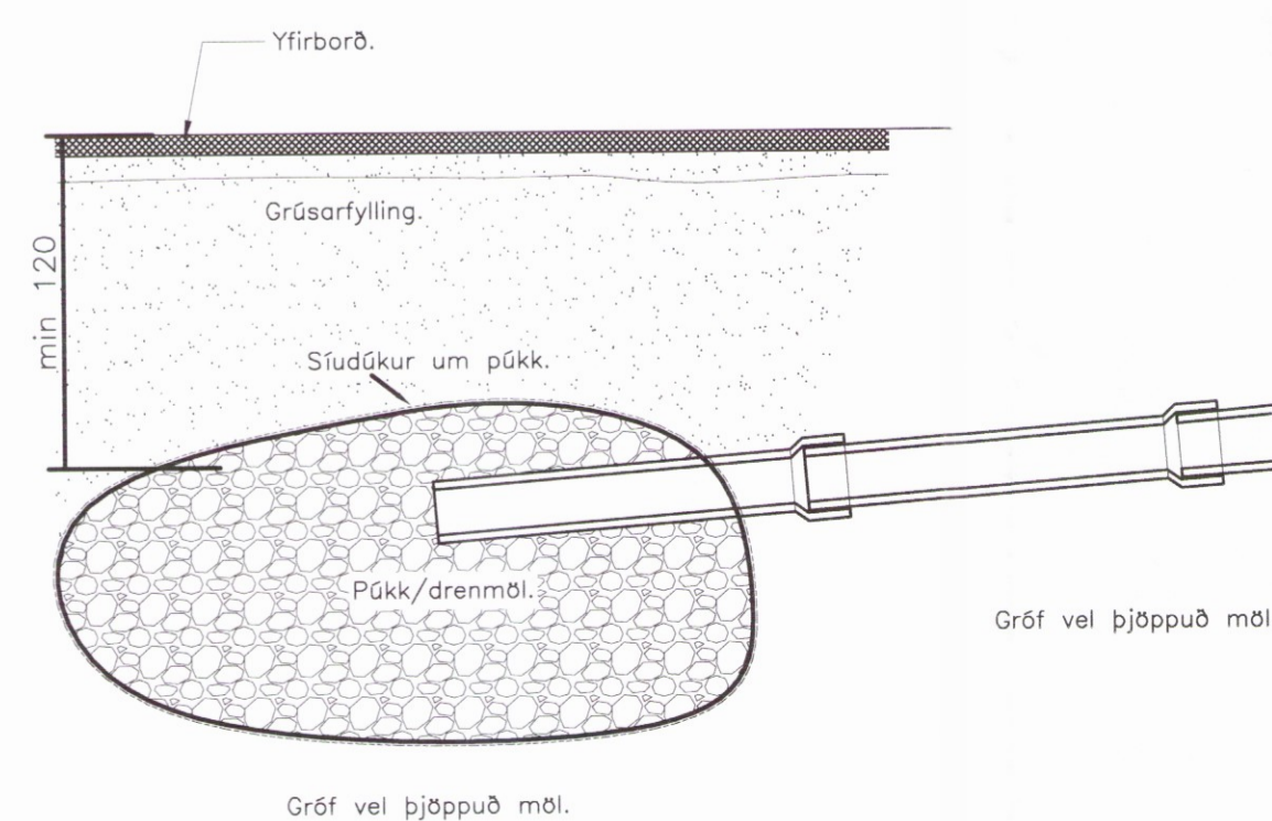
Sérmynd af púkki. 1:20.
