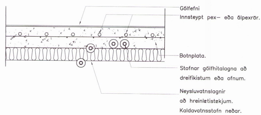
Snið í gólf. 1:10
