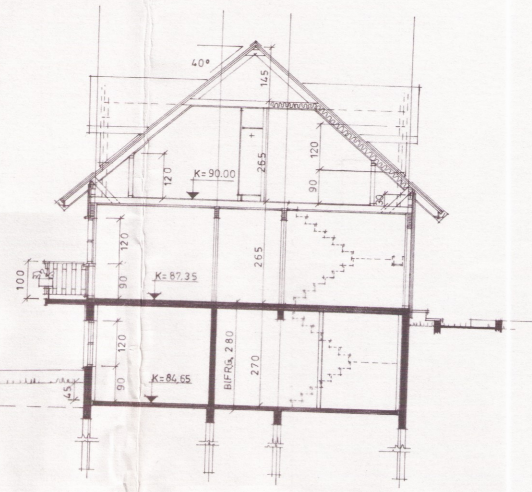
SNID A-A
