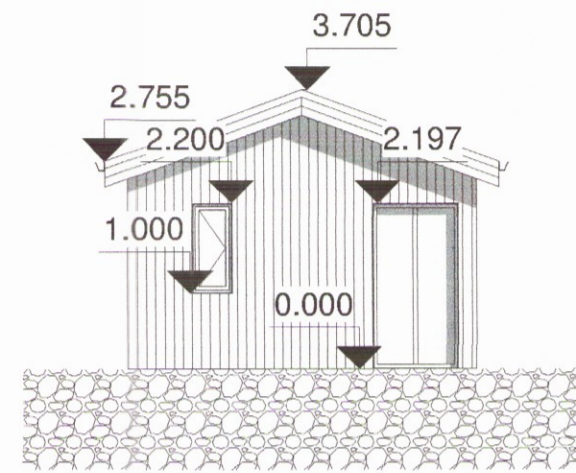
Vestlæg hlið Aðalupp útlit Mhl. 2 1 : 100
