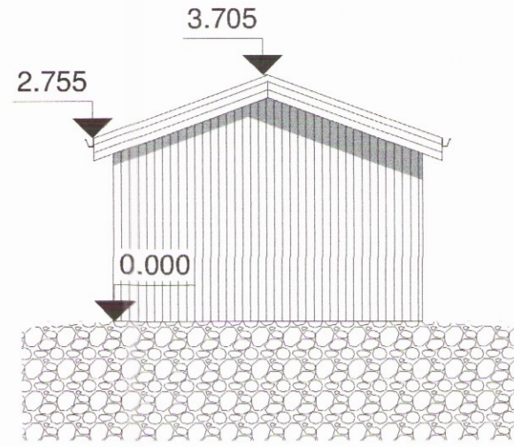
Austlæg hlið Aðalupp útlit Mhl. 2 1 : 100
