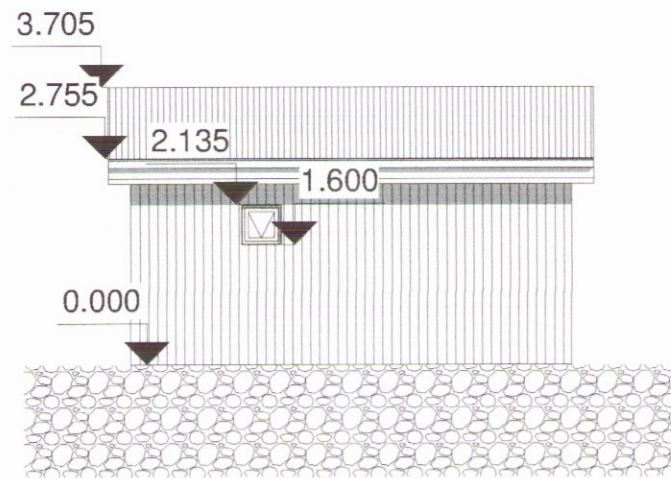
Norðlæg hlið Aðalupp útlit Mhl. 2 1 : 100
