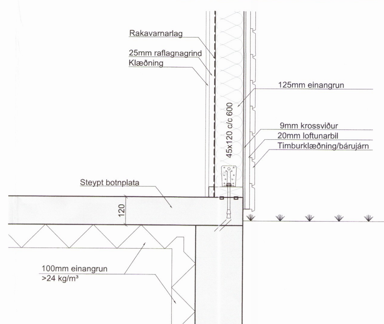
Deili - Veggir og sökkull Mkv. 1:10
