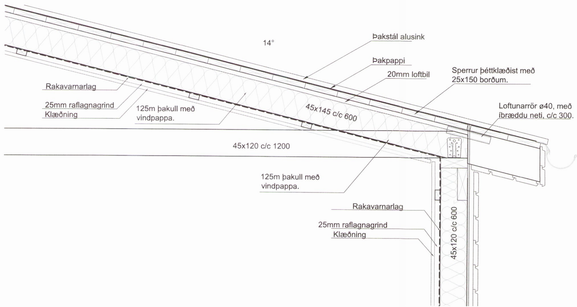
Deili - Þak og veggir Mkv. 1:10
