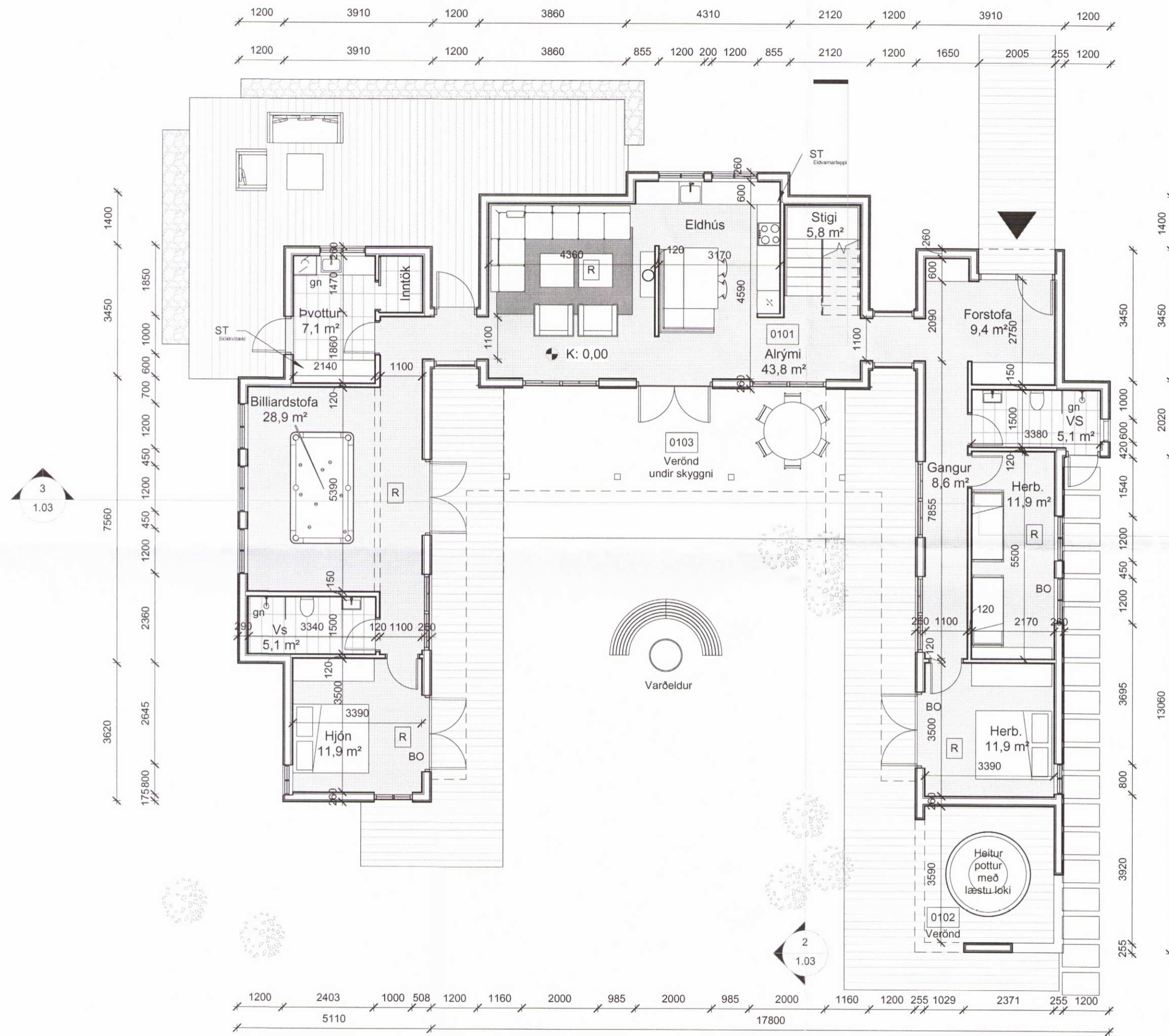
Grunnmynd 1.hæð 1 : 100
