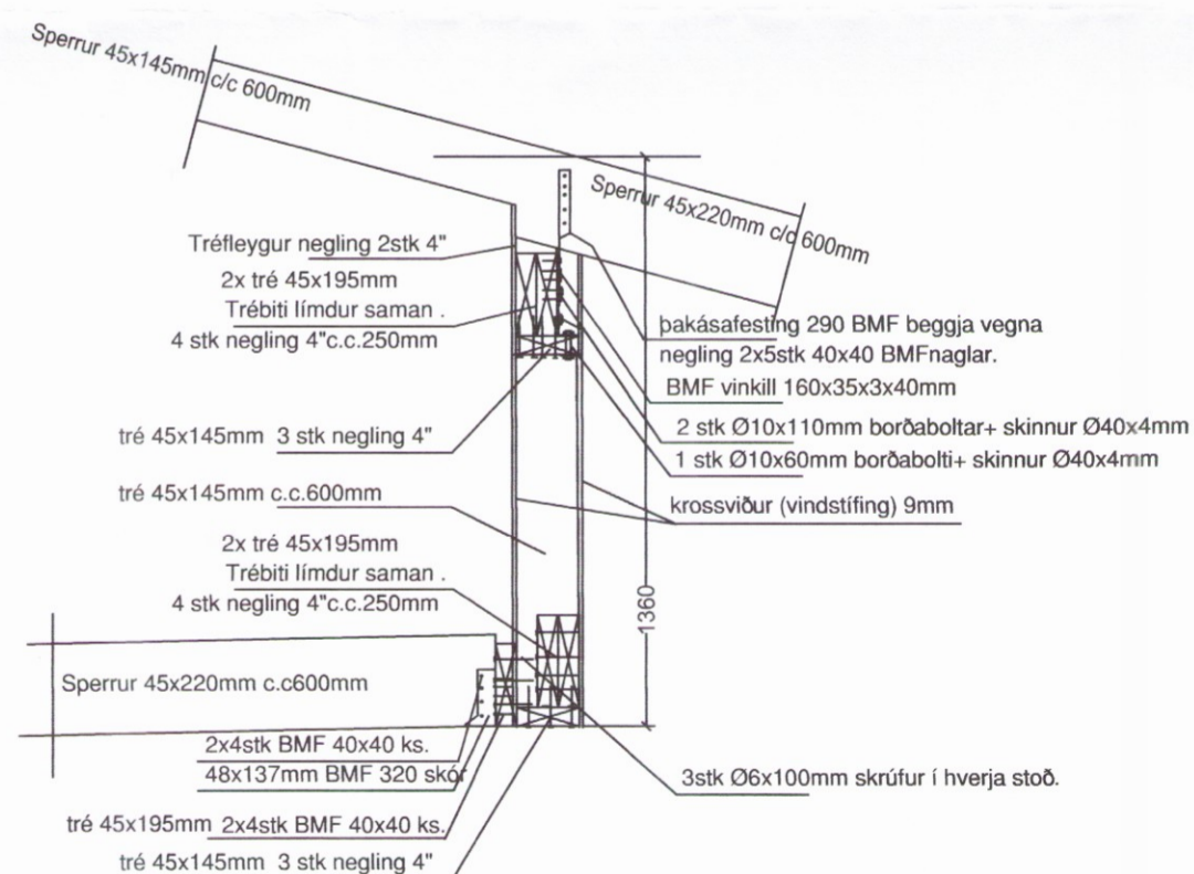
Snið Þ2 1:20
