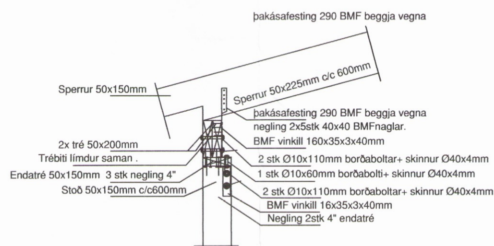
Snið Þ4 1:20
