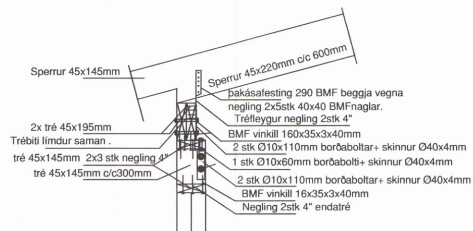
Snið Þ3 1:20
