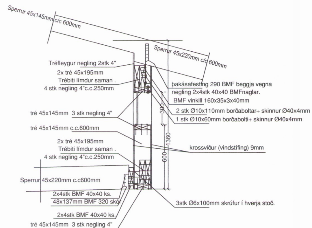
Snið Þ1 1:20
