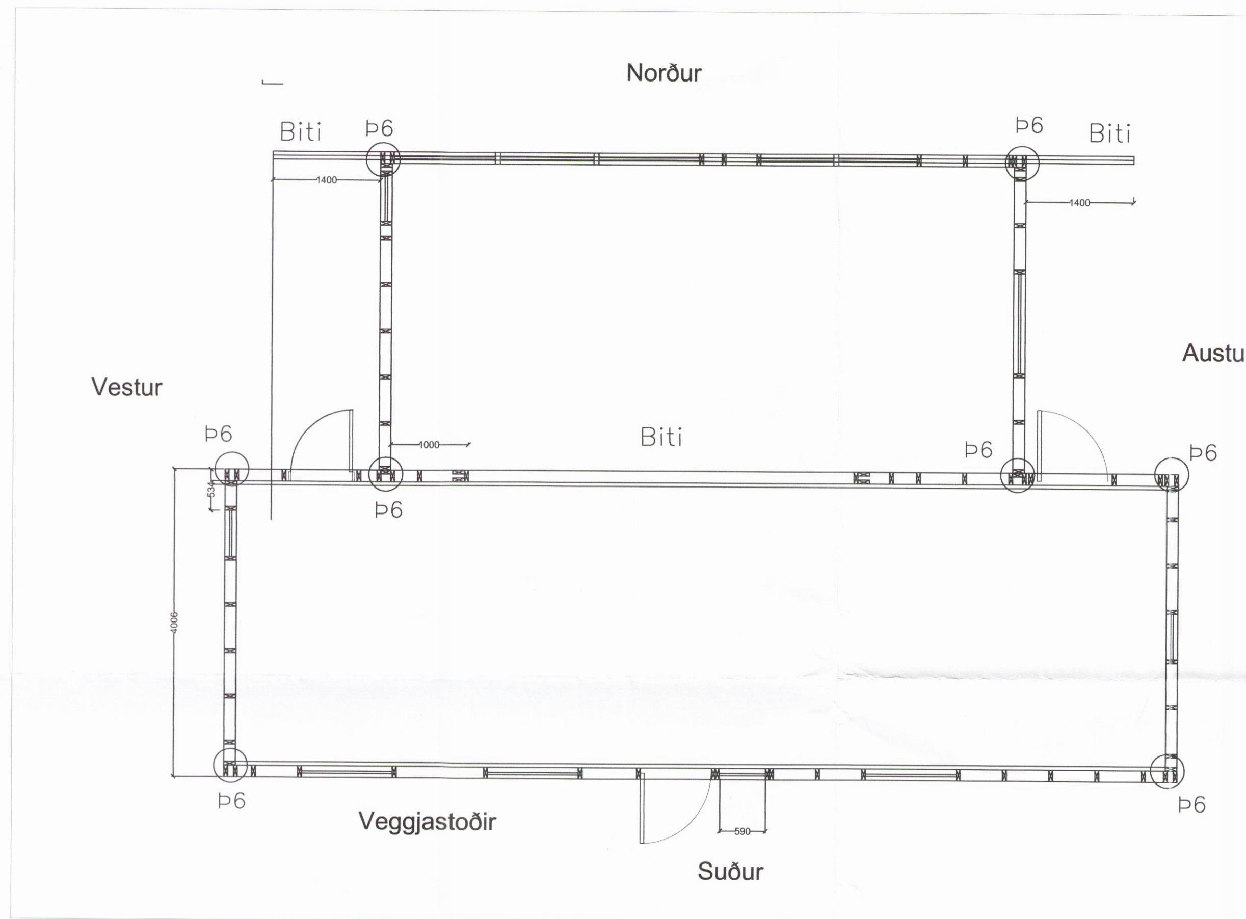
Grunnmynd Mkv. 1:50
