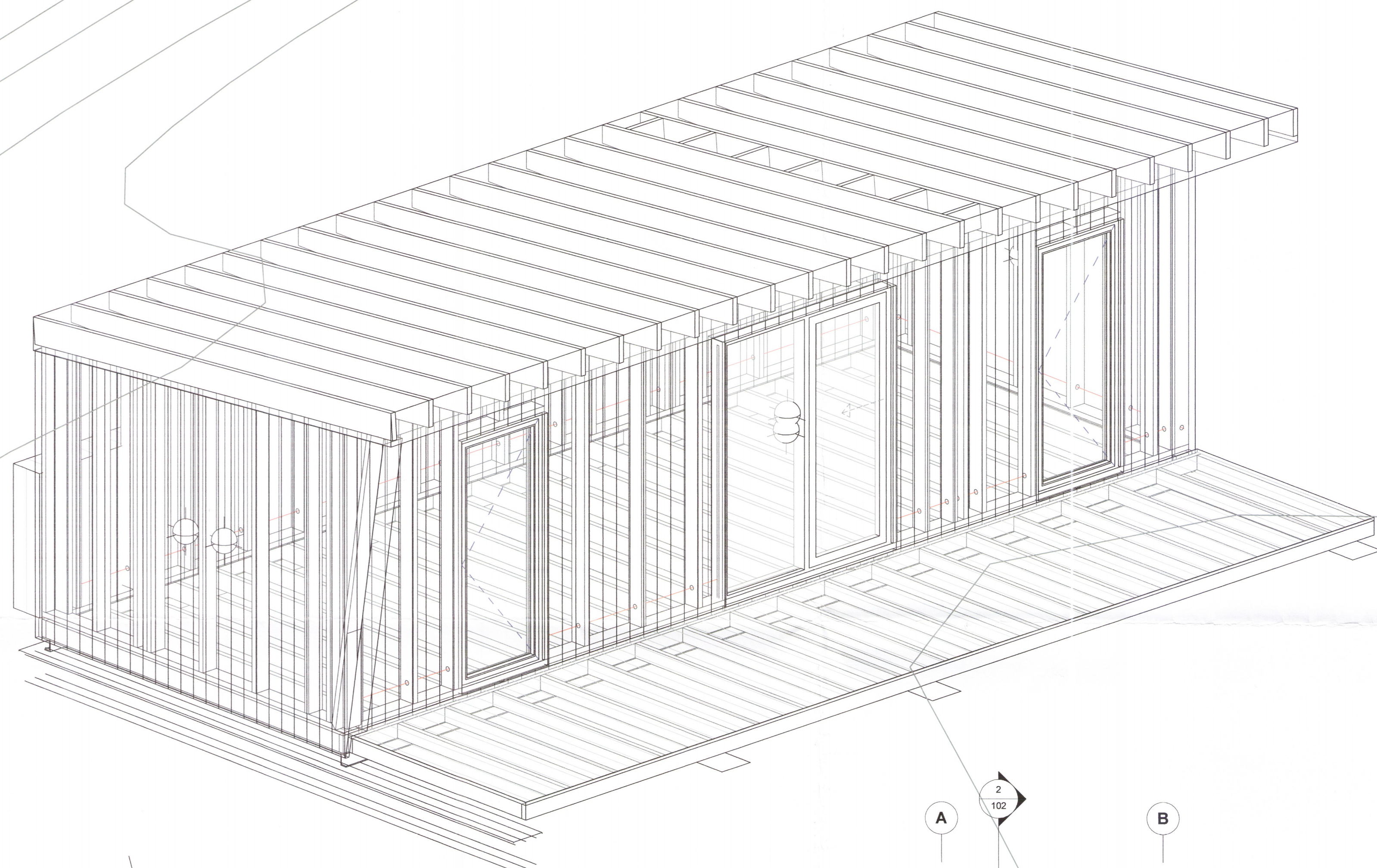
1 3D ásýnd burðargrinda
