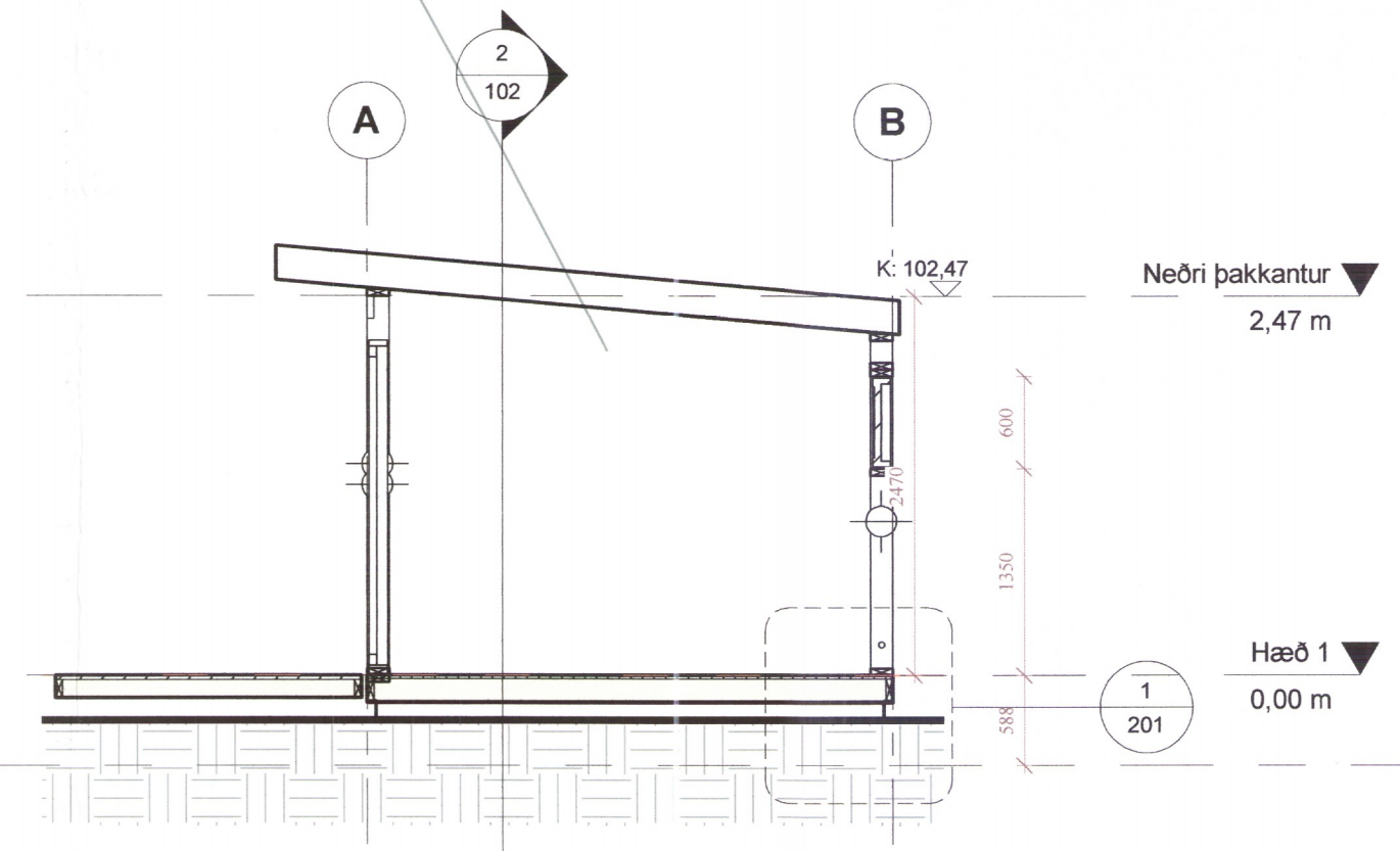
2 ÞVERSKURÐUR SÉRUPPDRÁTTUR 1 : 50
