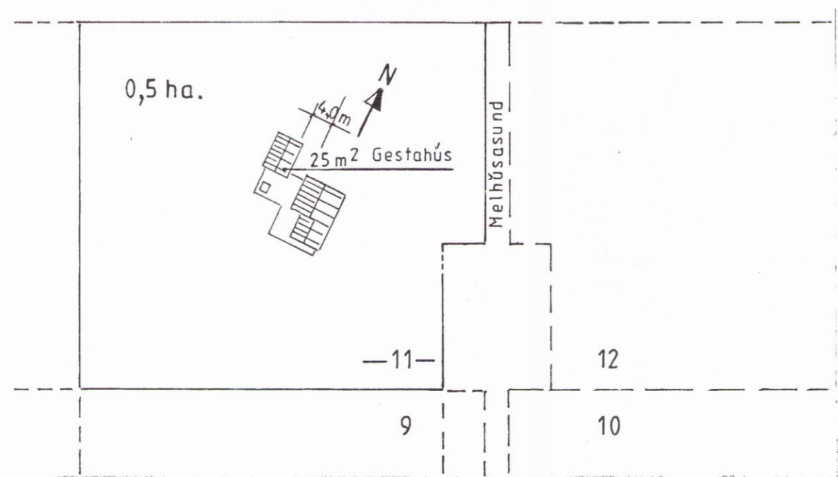
Afstöðumynd 1:1000
