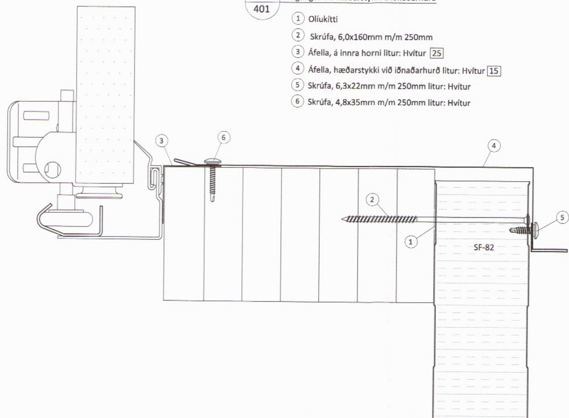
12 Frágangur við hæðarstykki á iðnaðarhurð 401
