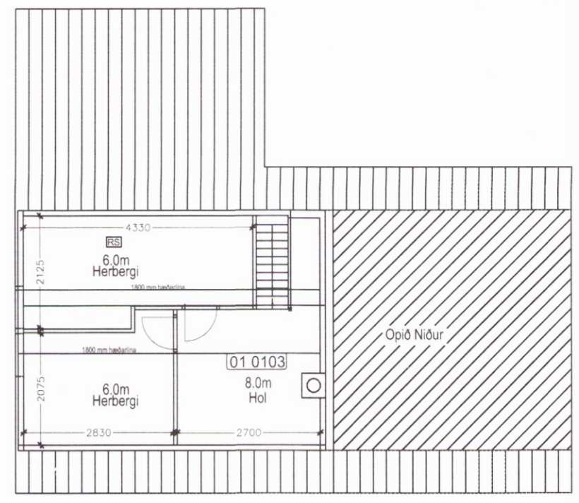
Grunnmynd Ris Mkv 1:100
