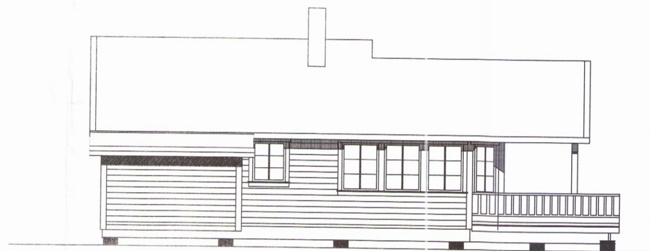
Ásýnd austurhlíðar Mkv 1:100
