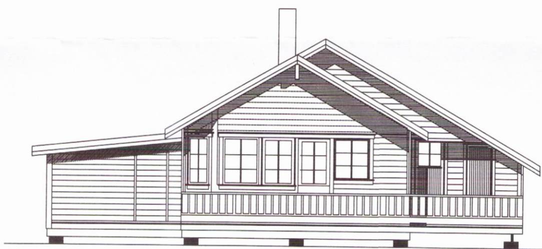
Ásýnd suðurhlíðar Mkv 1:100
