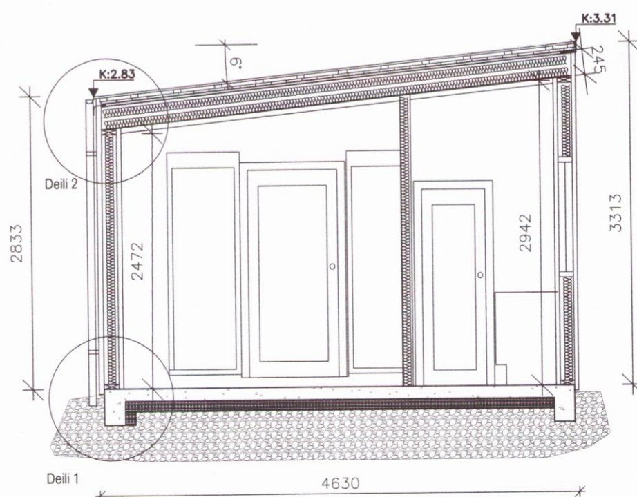
SNID A-A 1:50
