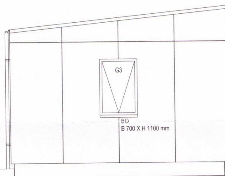
NORÐUR 1:50
