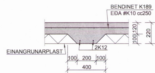
DEILI E 1:20
