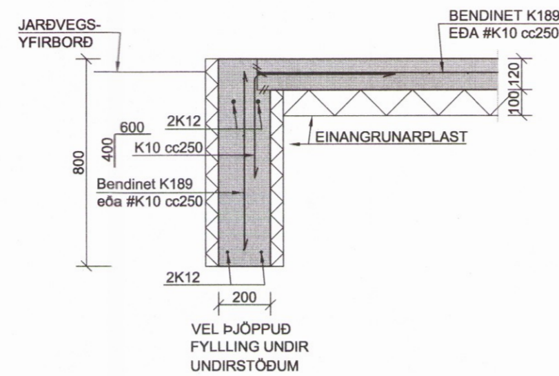
DEILI B 1:20
