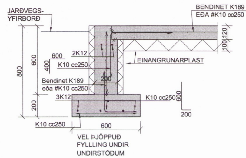
DEILI A 1:20
