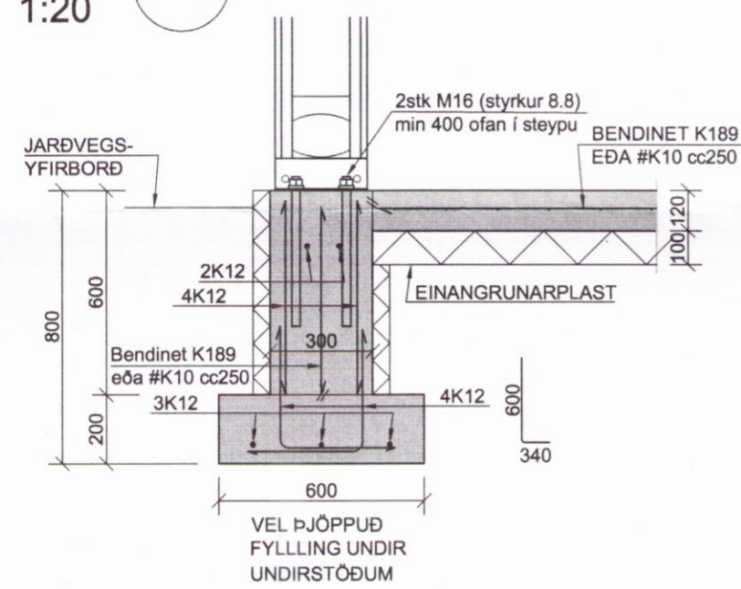
DEILI D 1:20
