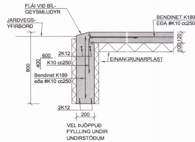
DEILI C 1:20
