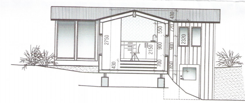
SNIÐ B-B MKV. 1:100
