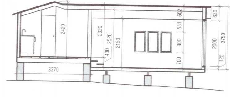
SNIÐ A-A MKV. 1:100
