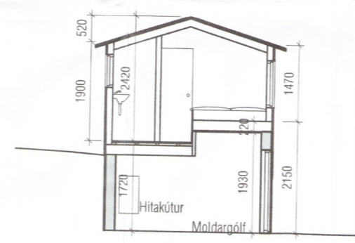
SNIÐ C-C MKV. 1:100
