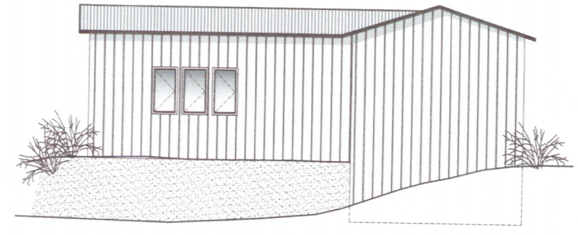
NORÐAUSTUR ÚTLIT MKV. 1:100
