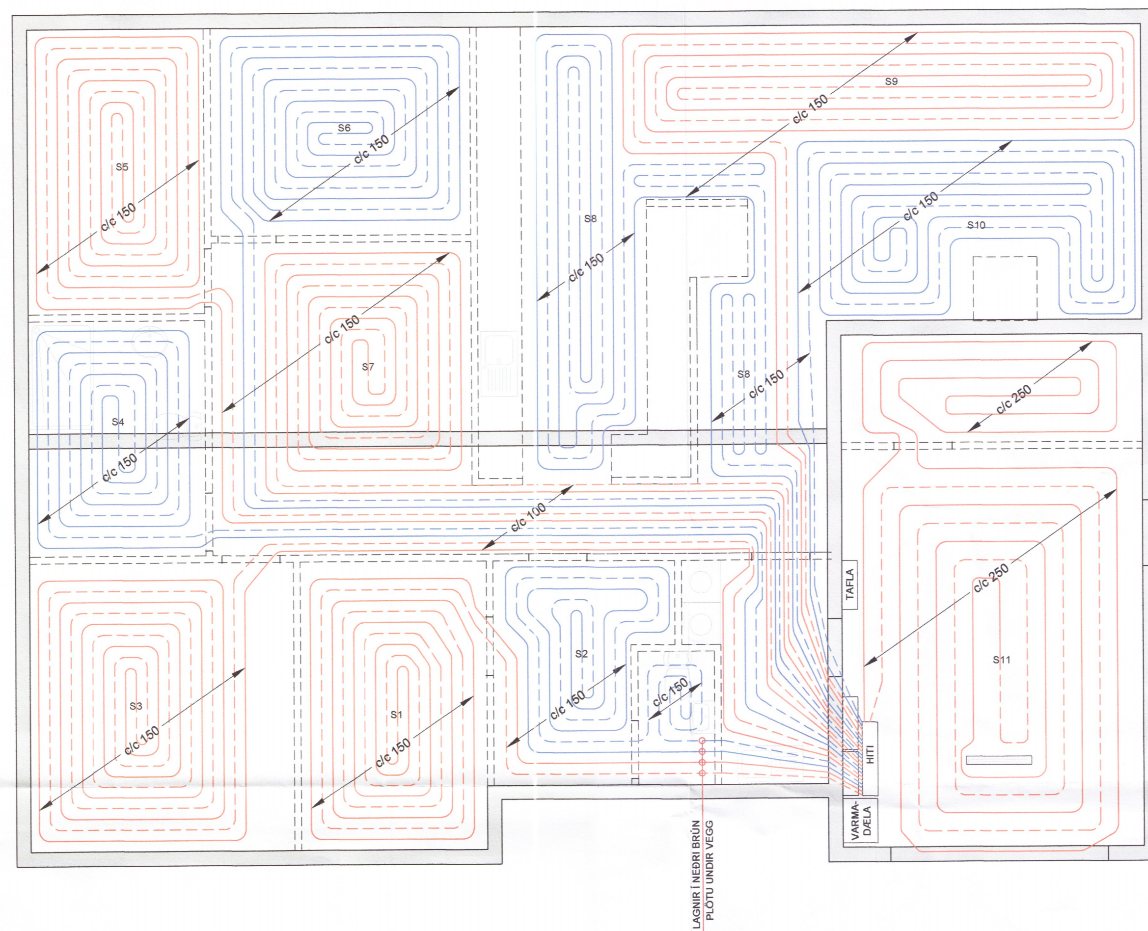
GRUNNMYND Mkv. 1:50
