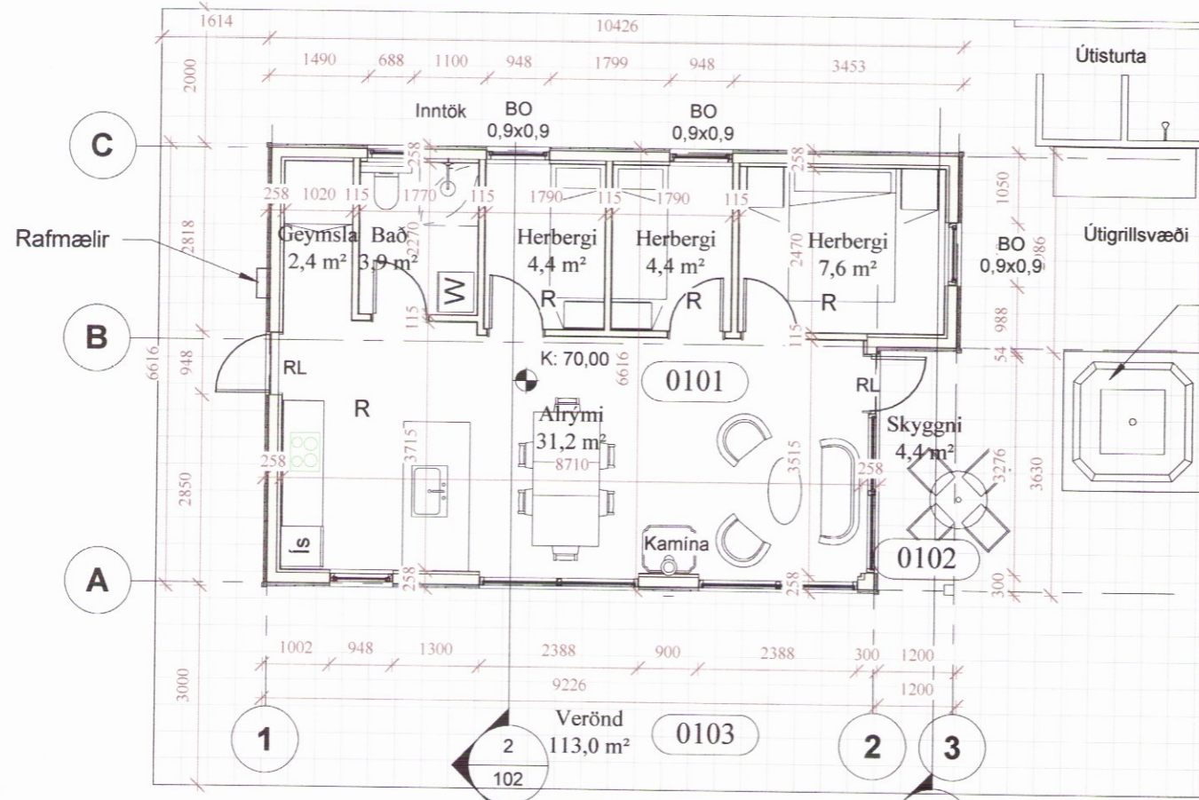
1 GRUNNMYND 1 : 100
