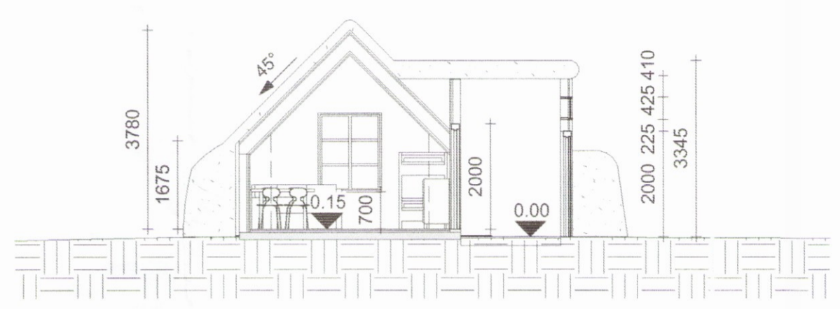
Snið A 1 : 100
