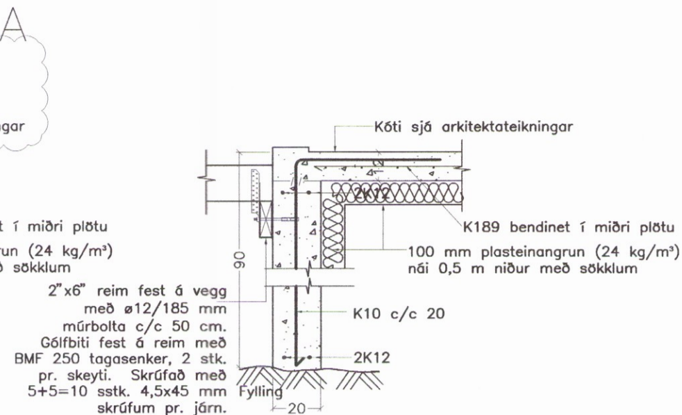
B SNID B-B. 1:20.
