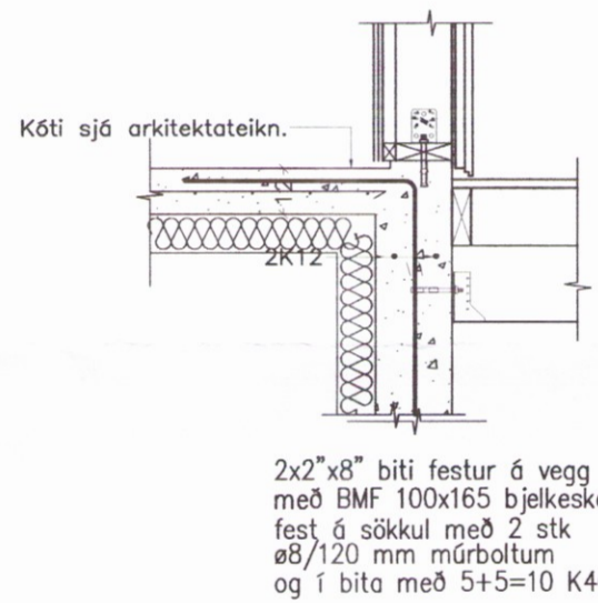
0.1 Sérmynd 0.1 1:20.
