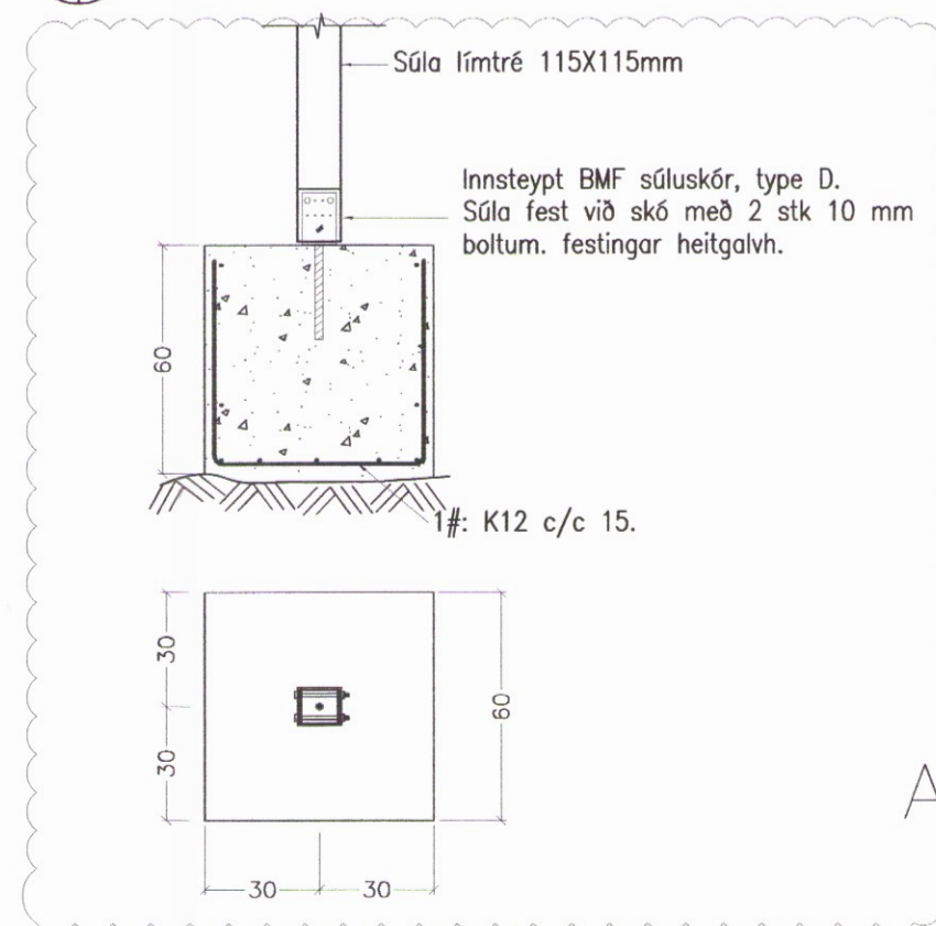
U2 Undirstaða U2. 1:20.
