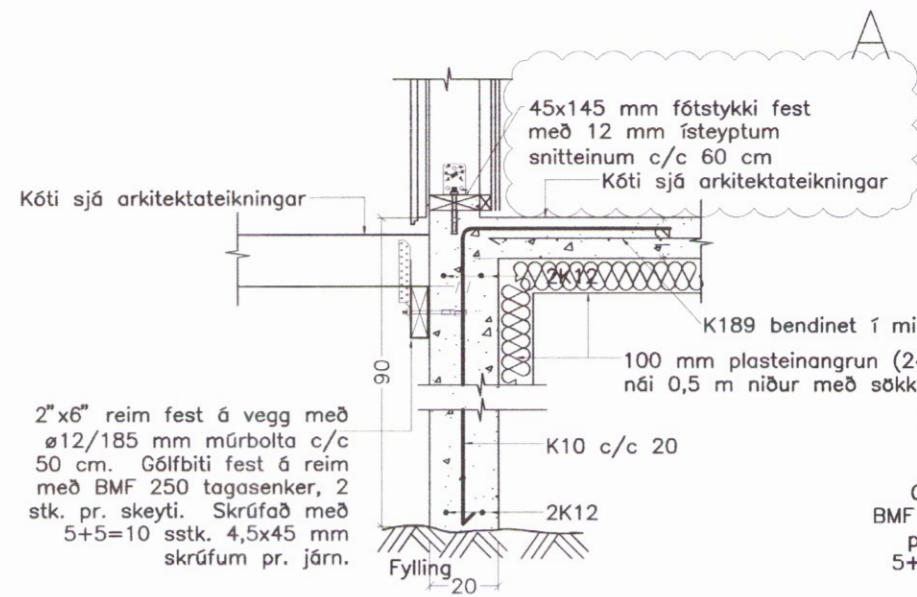
A SNID A-A. 1:20.
