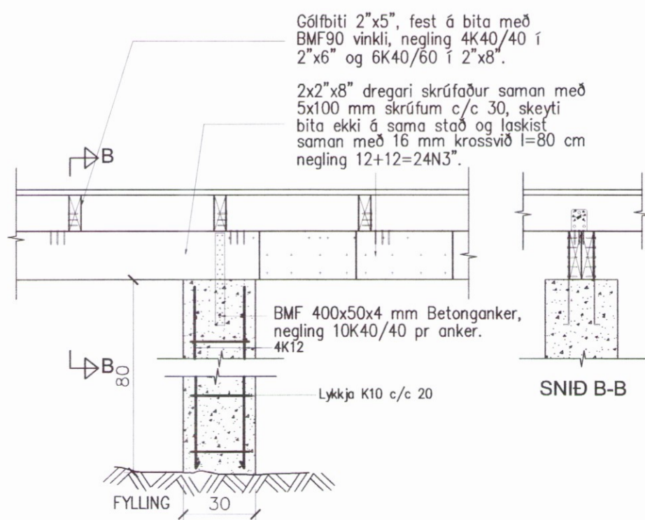
U1 Undirstaða U1. 1:20.
