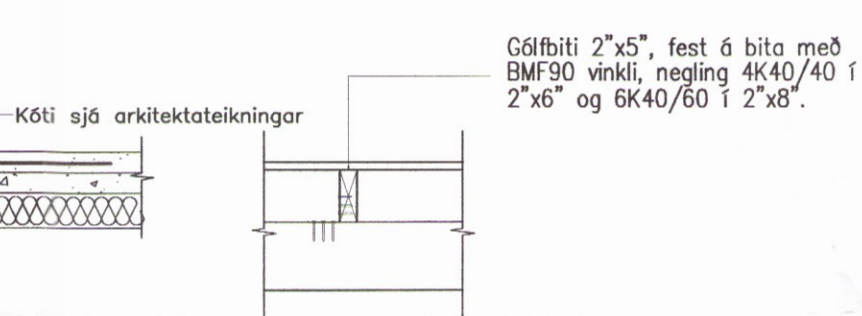
0.3 Sérmynd 0.3 1:20.
