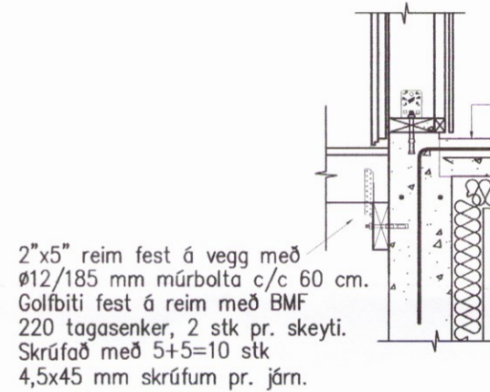
0.1 Sérmynd 0.1 1:20.
