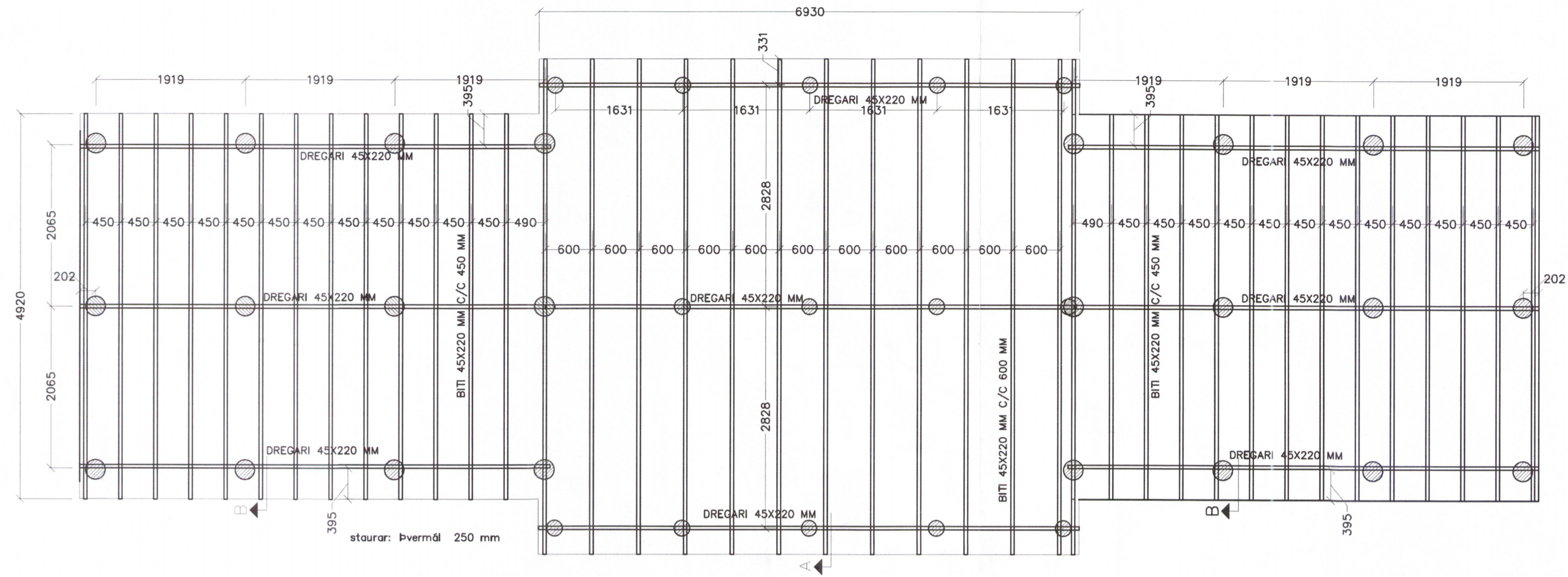
GRUNNMYND UDIRSTÖÐUR 1:50
