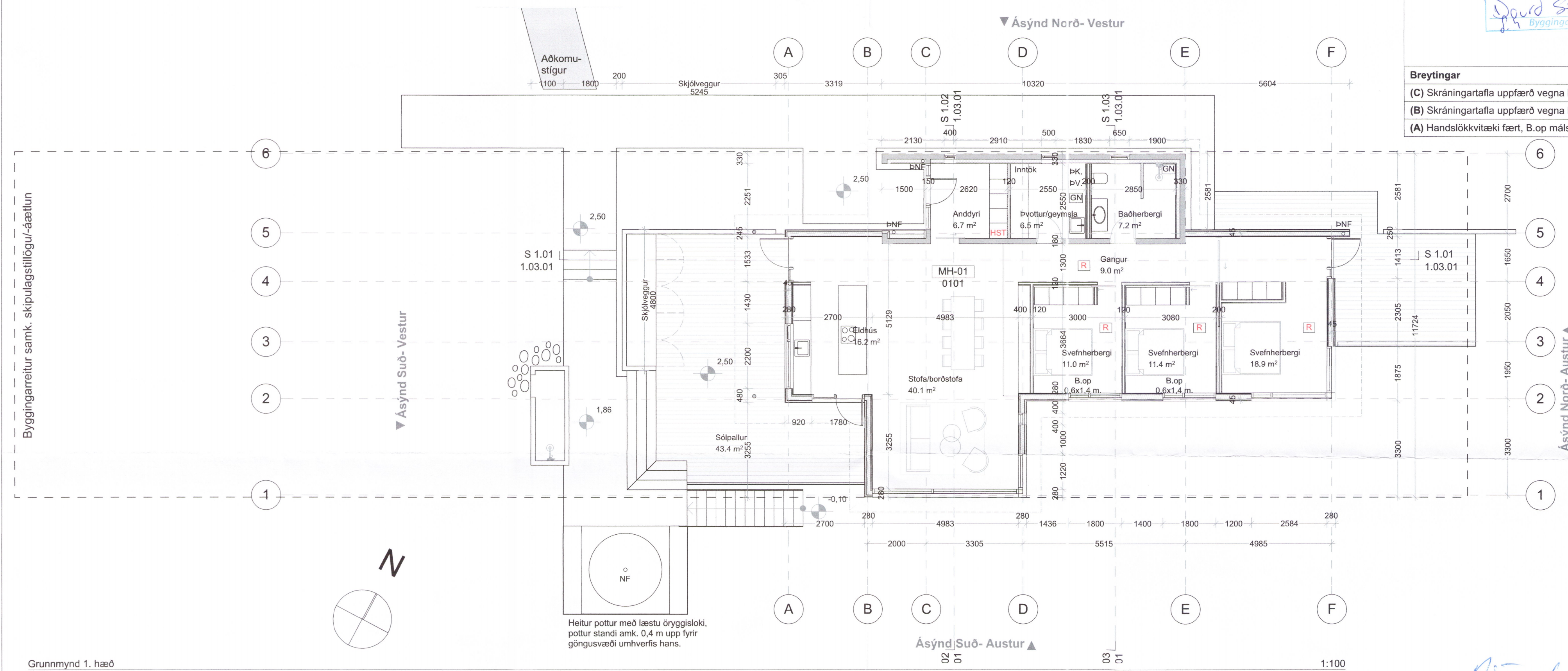
Grunnmynd 1. hæð
