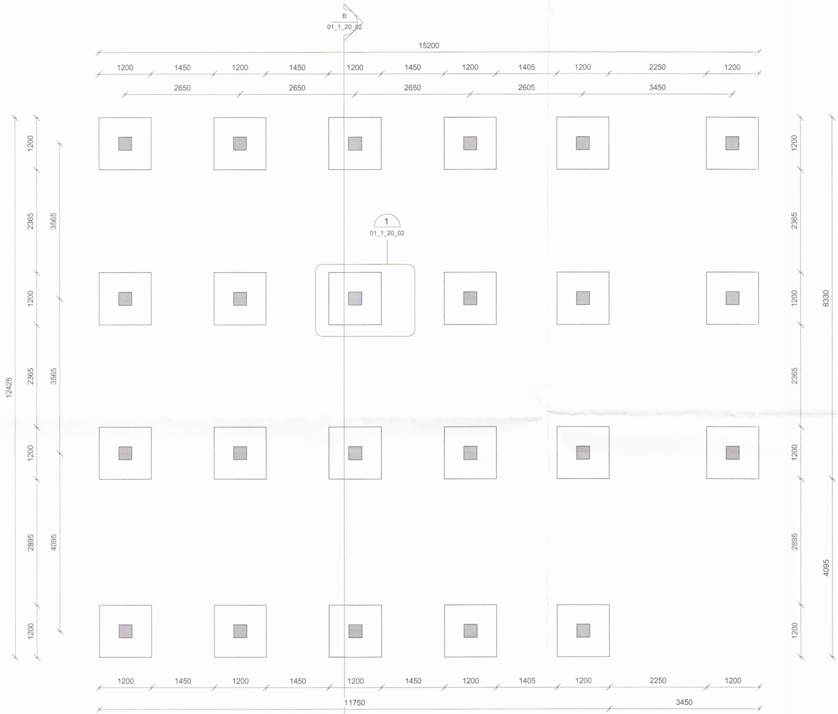
Grunnmynd undirstaða 1 : 50
