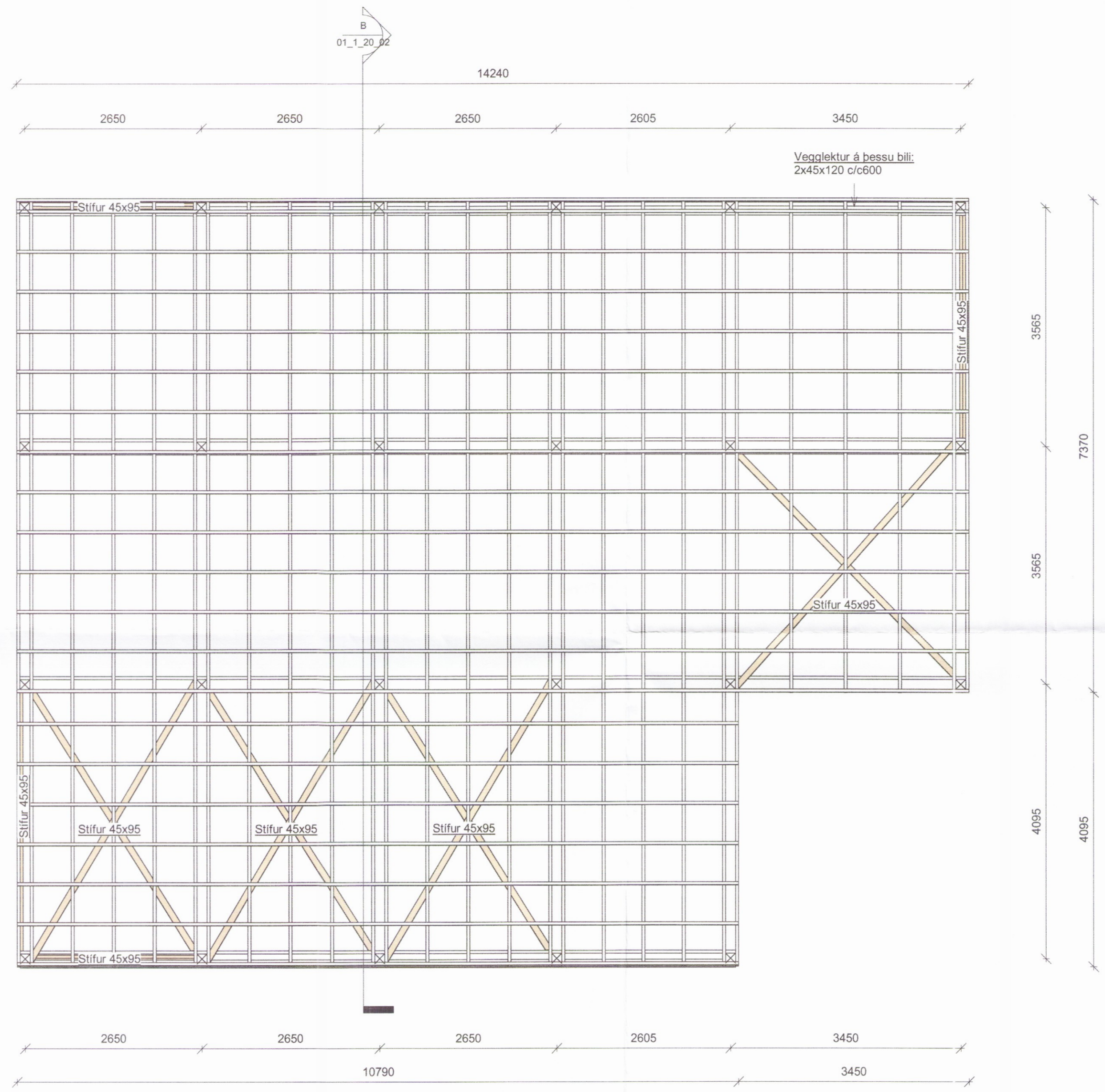
Grunnmynd timburvirkis 1 : 50
