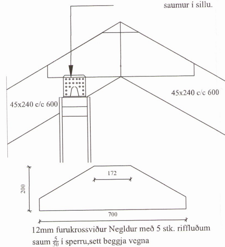
08 Snið 08 Mk. 1:10
