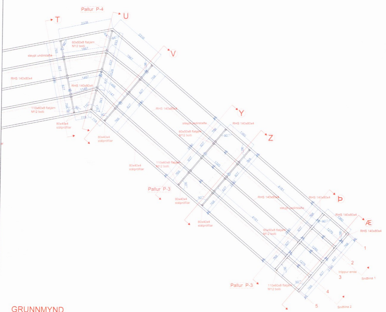
GRUNNMYND
