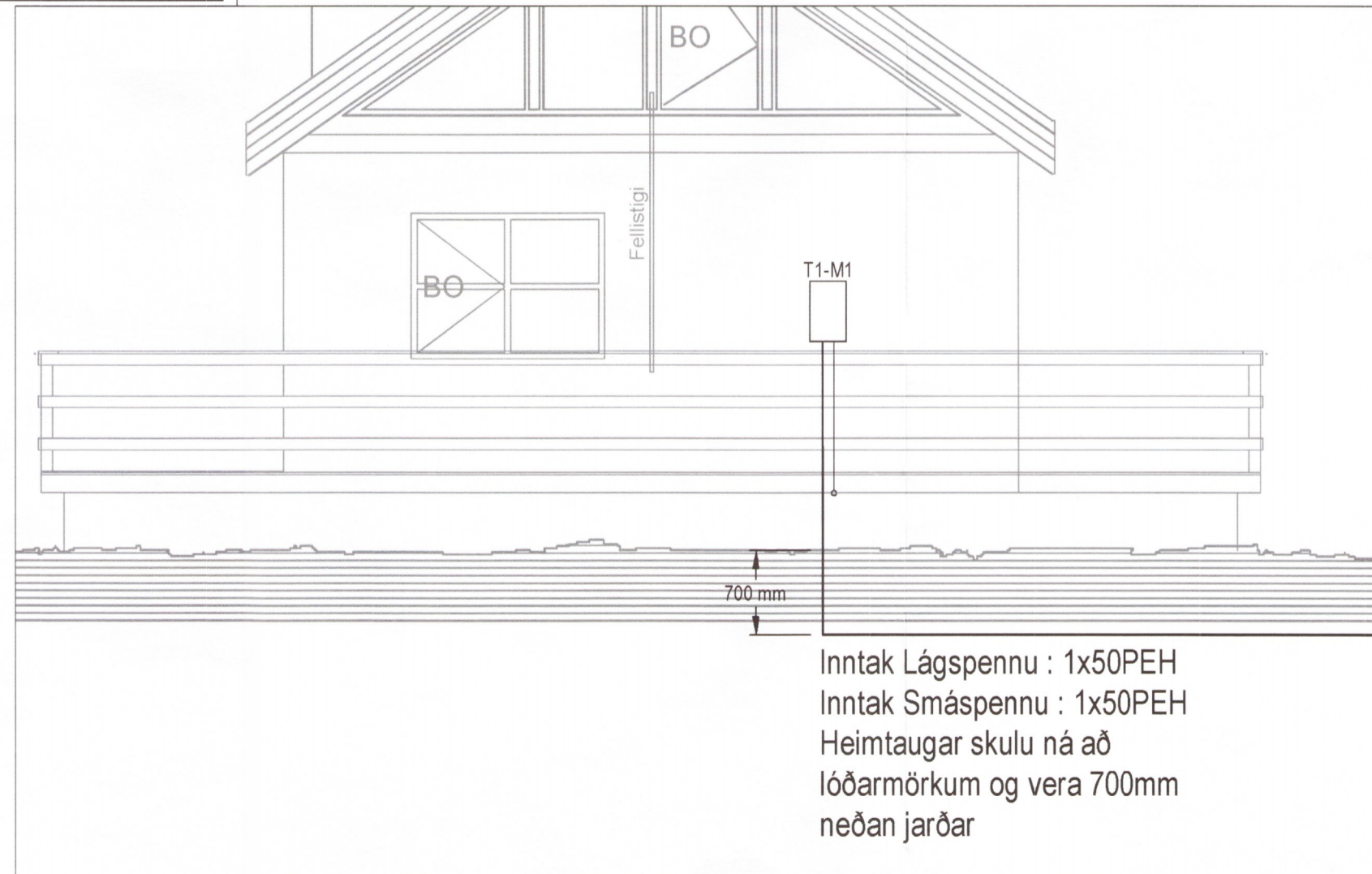
Snið A 1:50
