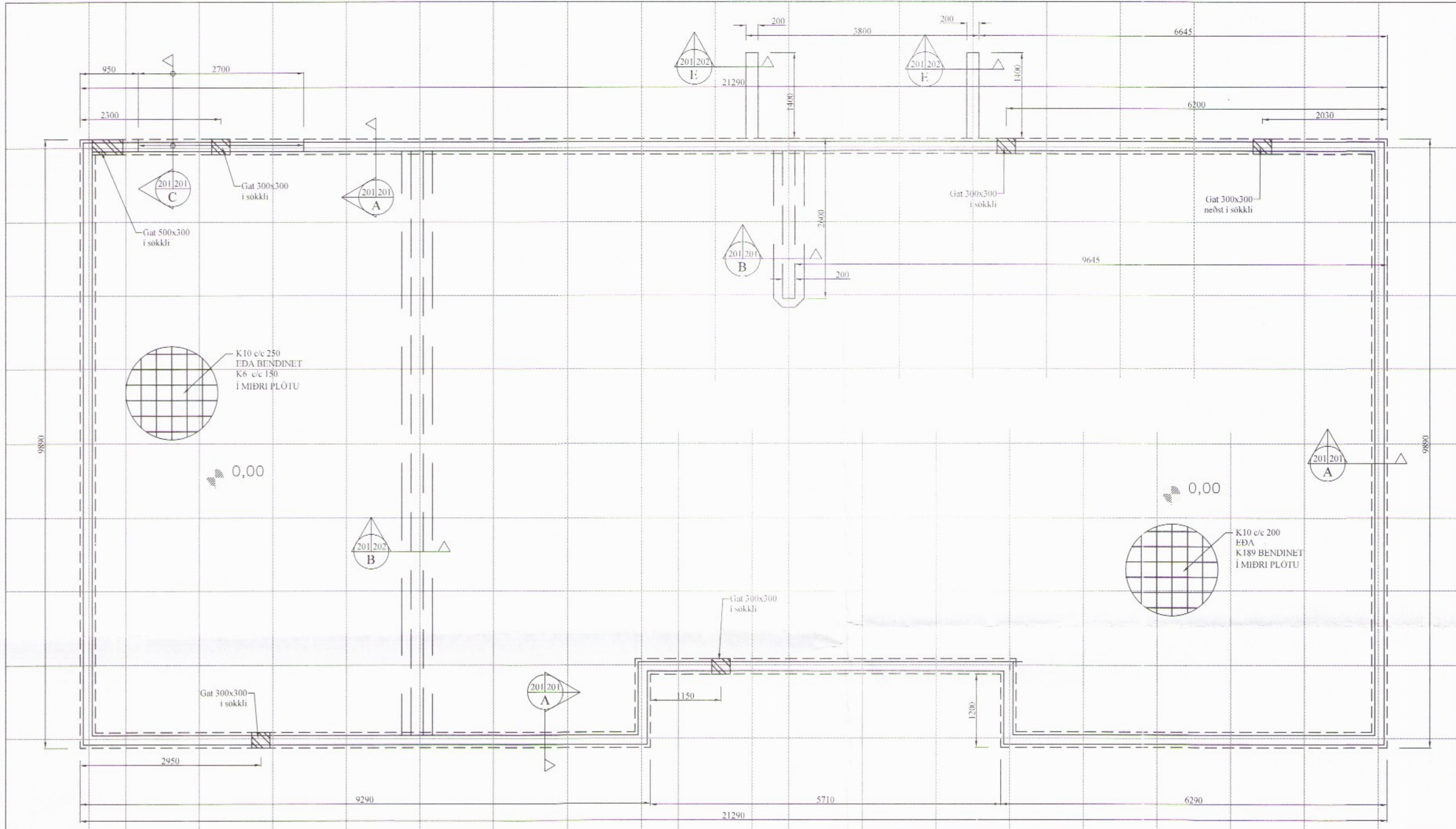
GRUNNMYND SÖKKULS Mkv. 1:50
