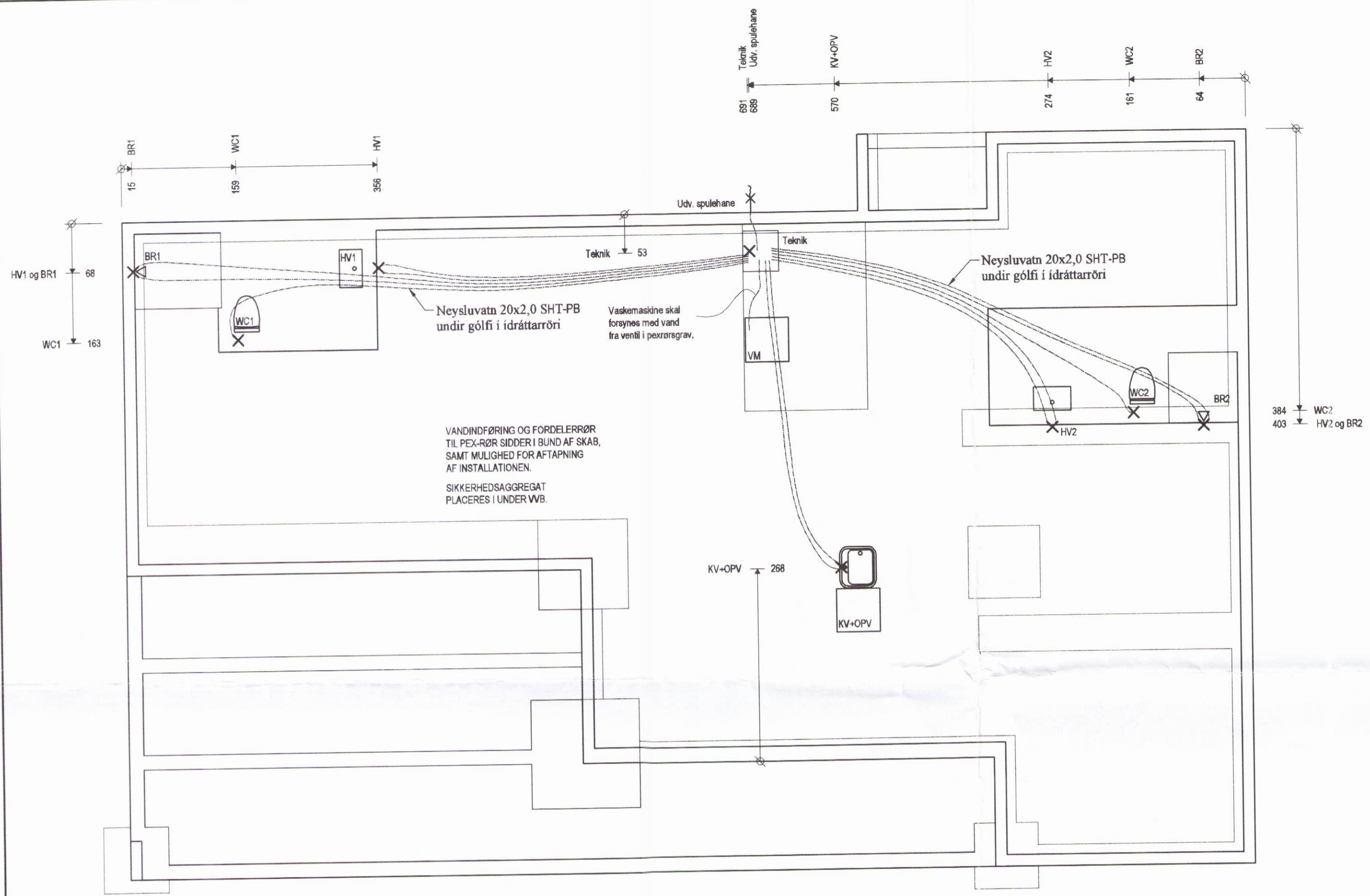
Neysluvatnslagnir, Grunnmynd, 1:50
