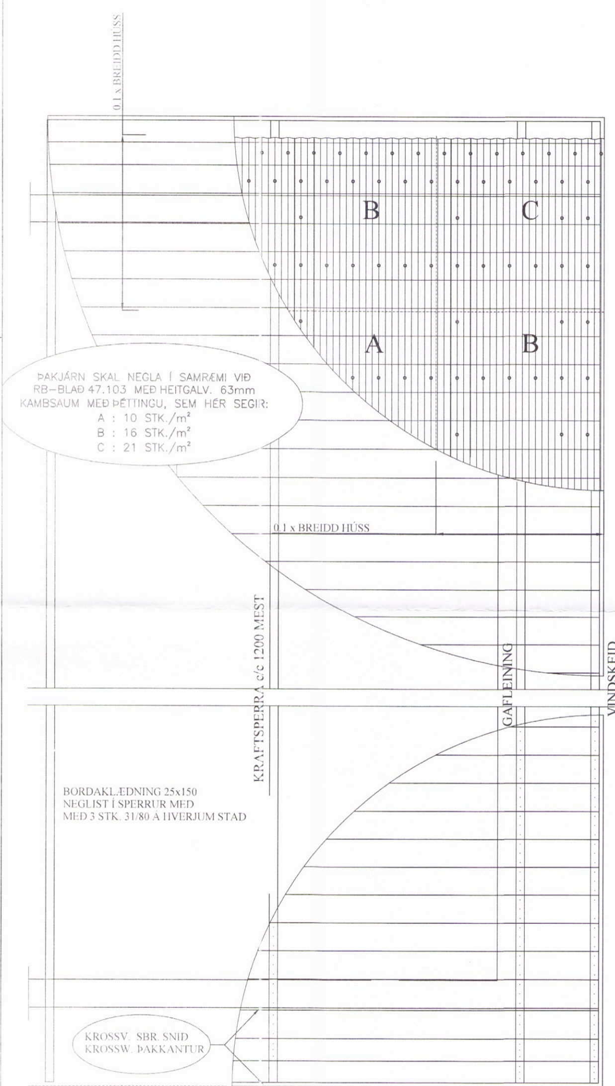
NEGLING ÞAKKLÆÐNINGAR MKV. 1:20
