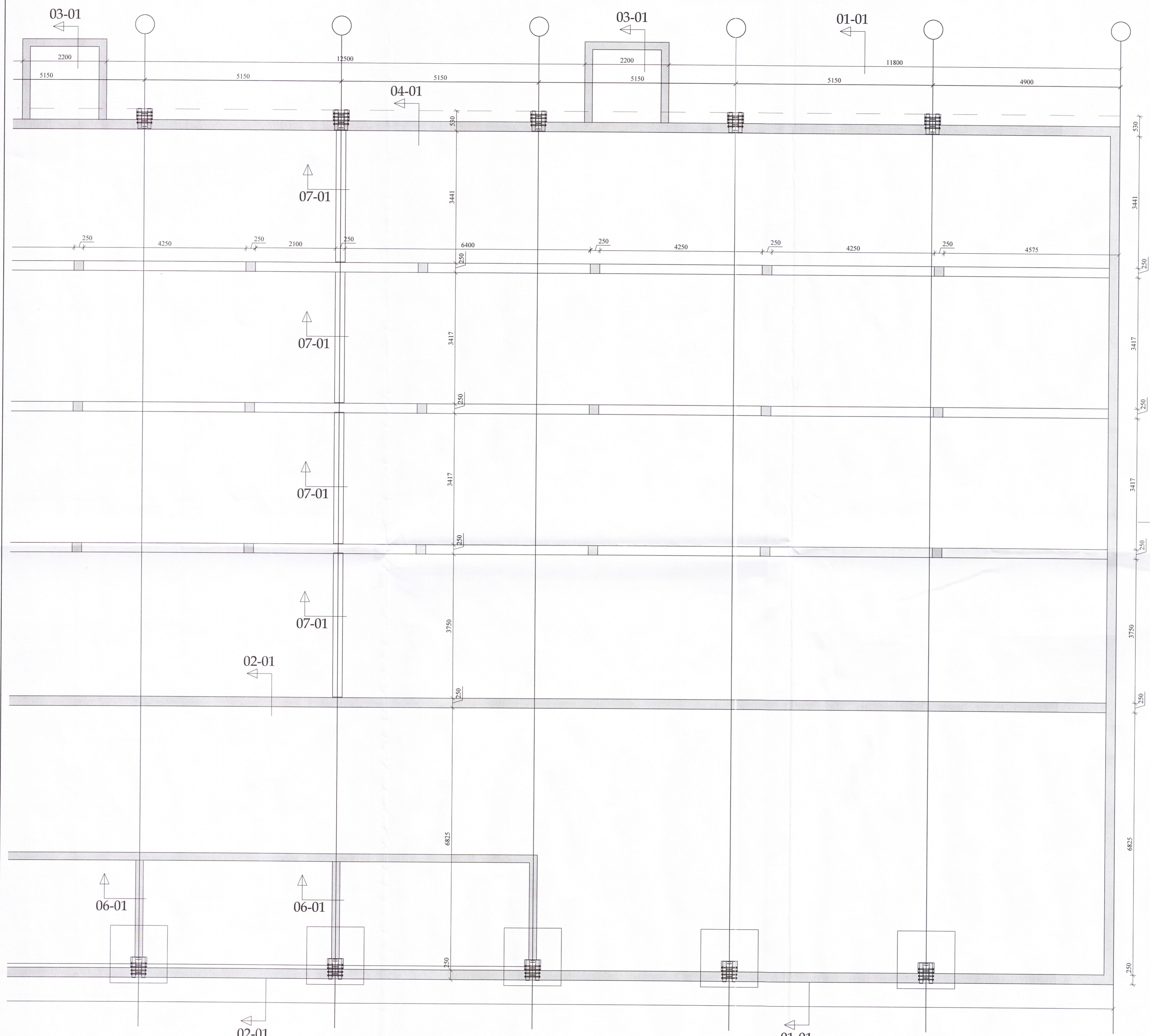
Grunnmýnd kjallara að hluta mk. 1:50
