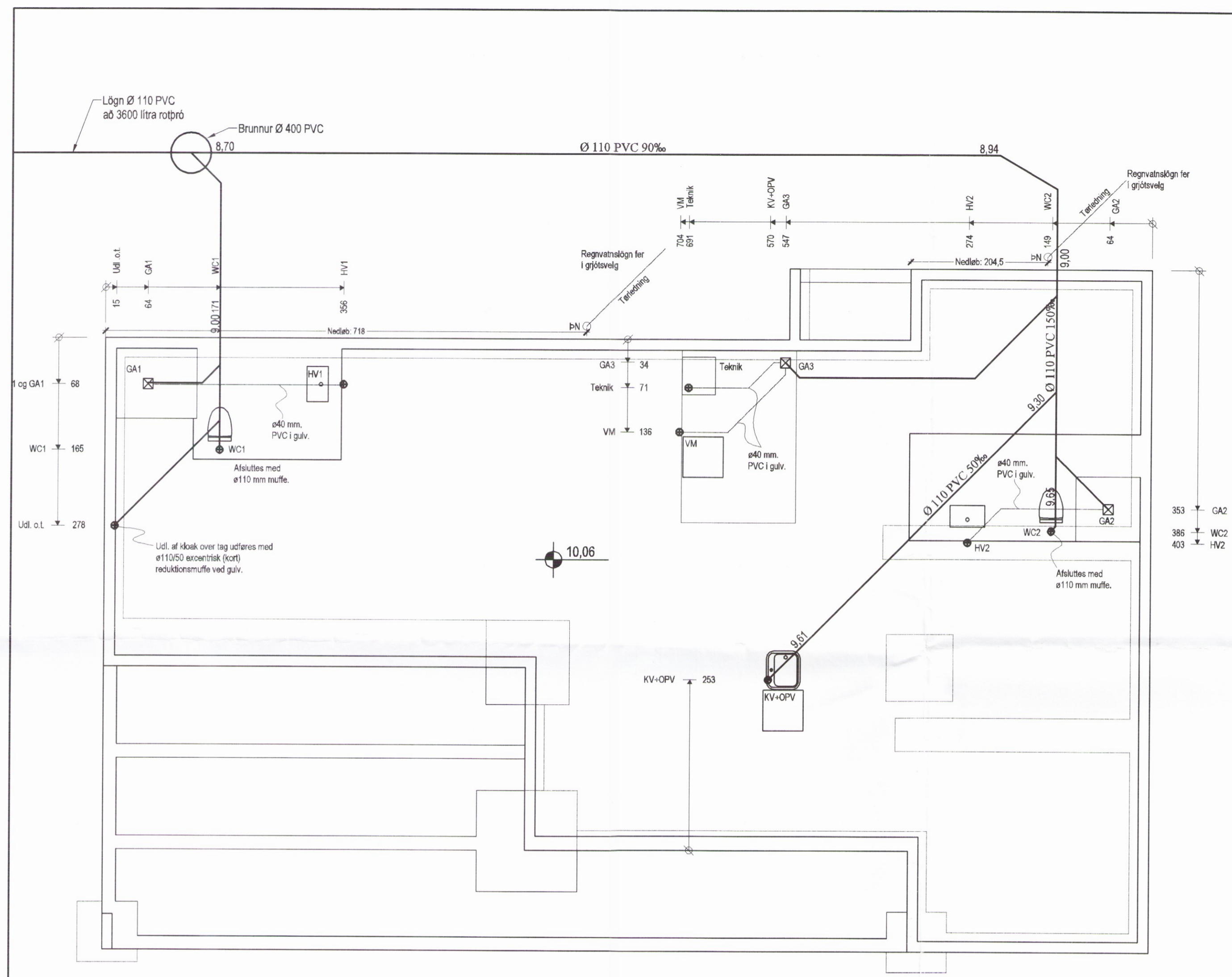
Fráveitulagnir, Grunnmynd, 1:50
