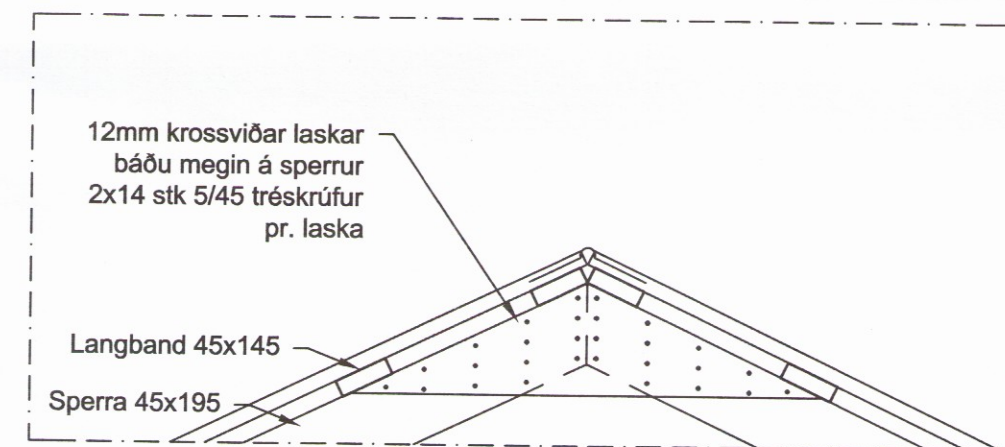
07 DEILI 1:20
