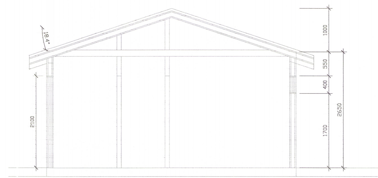
SNIDMYND A-A.
